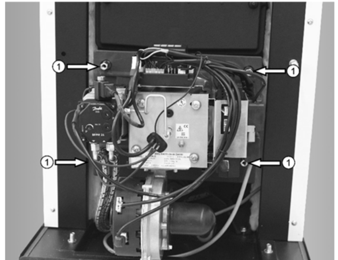
Abb. 64: Muttern ① der unteren Kesseltür (Der abgebildete Brenner entspricht evtl. nicht dem gelieferten.)
