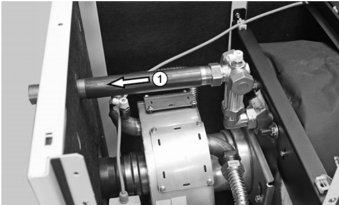
Abb. 14: Vorlauf Direktkreis ① (bei Standardausführung ecoDUO .. / ecoOEL Pro ..)
