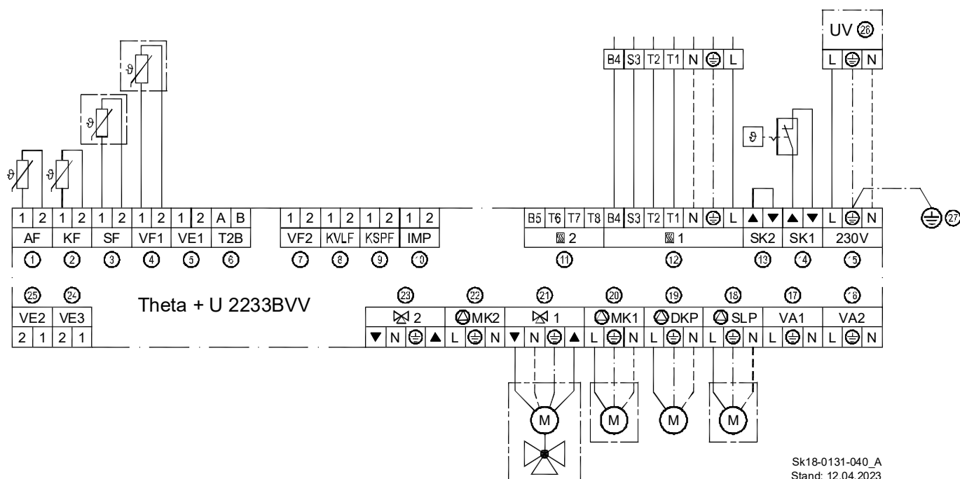
Abb. 26: Elektrische Anschlüsse und Stromlaufplan für ecoDUO... und ecoOEL Pro... (mit Raketenbrenner® RE .. HUG) sowie ecoDUO GAS... (mit Gas-Gebläsebrenner GE.. HUG)
