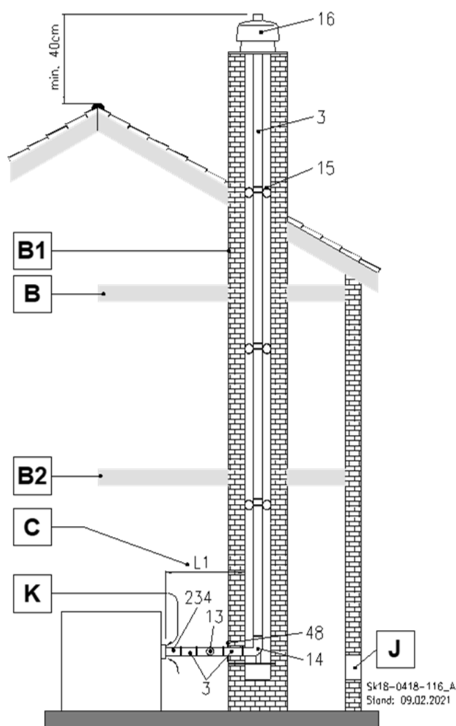
Abb. 29: B 23 Abgasrohr im Schornstein
