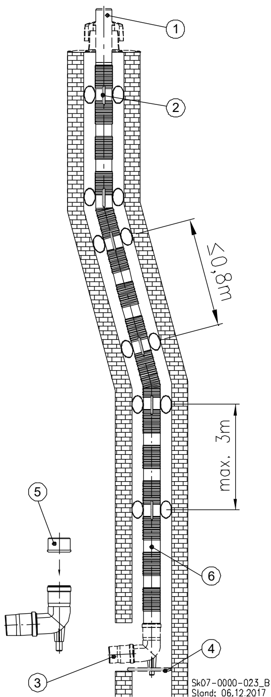
Abb. 45: Kaminsystem, flexibel
