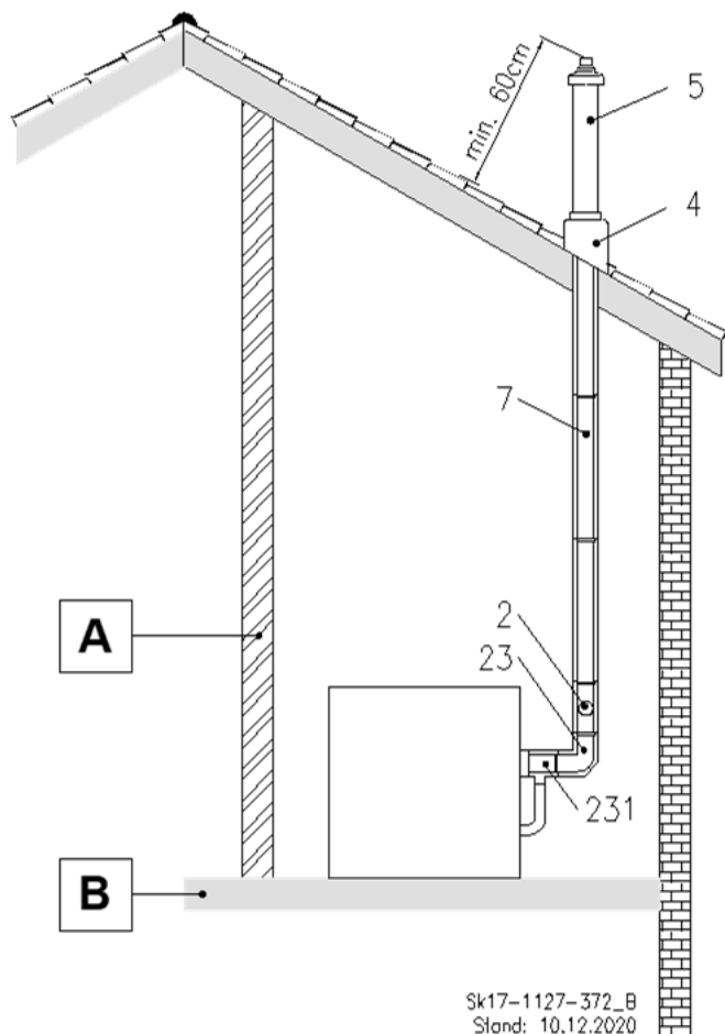
Abb. 33: C 33x Dachheizzentrale mit der Durchführung senkrecht durch ein Schrägdach
