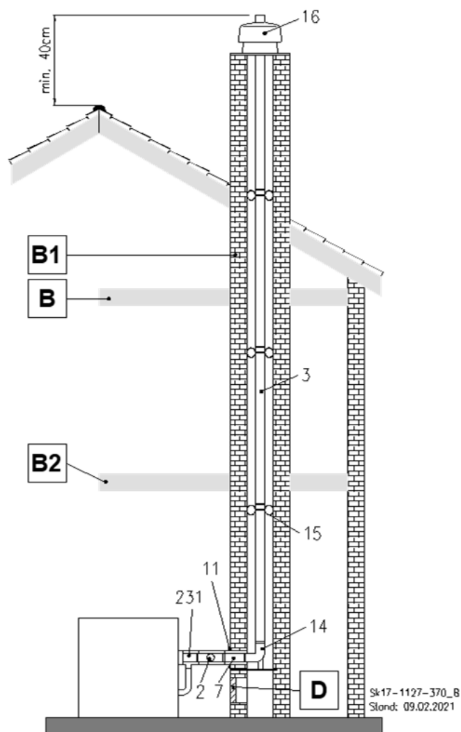
Abb. 38: C 93x Abgasrohr im Schacht
