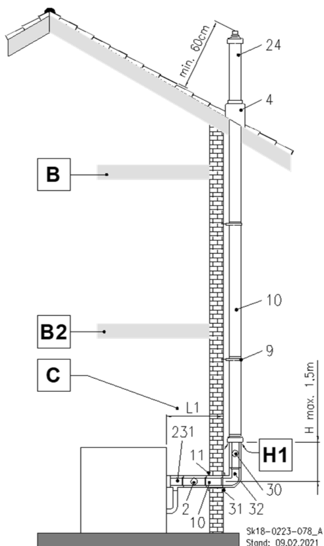
Abb. 34: C 53x Außenwandführung LAS
