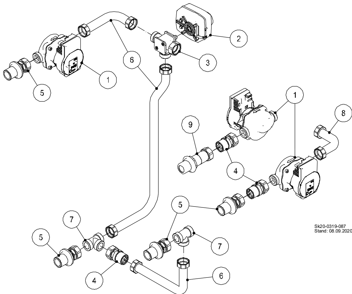
Abb. 77: Pumpen-, Mischerkreis und Speicherladeset
