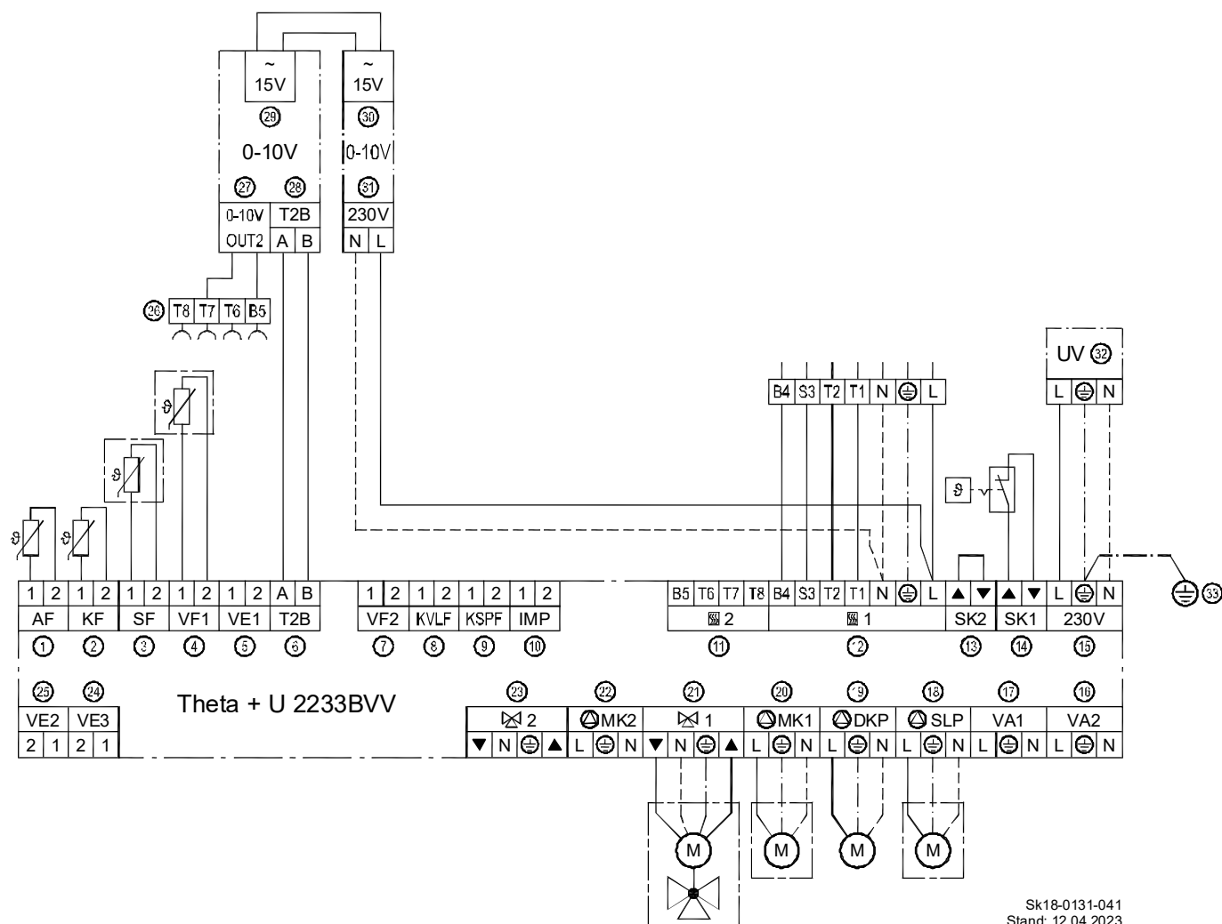
Abb. 25: Elektrische Anschlüsse und Stromlaufplan für ecoDUO...m (Raketenbrenner® RM .. EUG)
