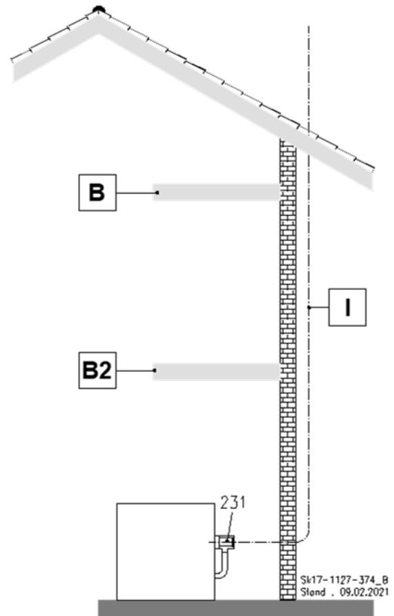
Abb. 35: C 63x Für Anschluss an eine nicht mit der Gasfeuerstätte geprüfte Verbrennungsluftzuführung und Abgasabführung
