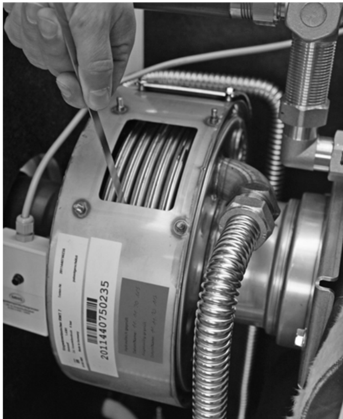
Abb. 71: Anwendung der Reinigungsklinge
