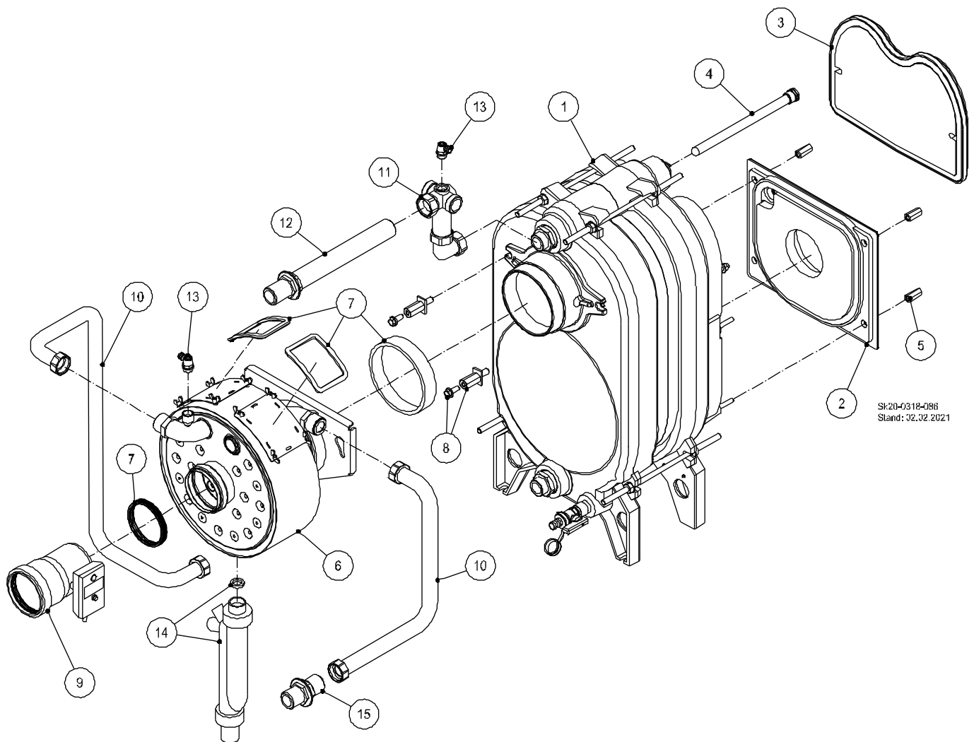
Abb. 76: Gussblock, RWT und Basis
