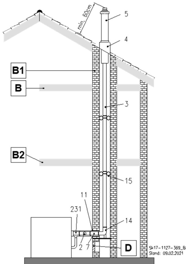
Abb. 37: C 93x Luft-Abgas-System im Schacht und Luft-Abgas-Rohrsystem mit Dachdurchführung
