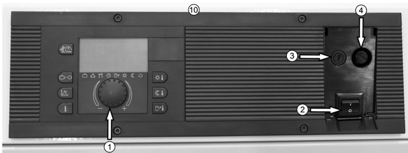
Abb. 79: Kesselschaltfeld
