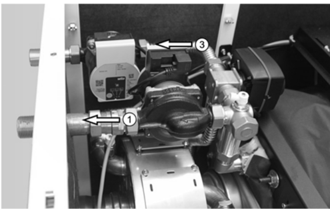
Abb. 15: Vorlauf Direktkreis ① sowie Vorlauf Mischerkreis ③ (bei Ausführung ecoDUO ..i)
