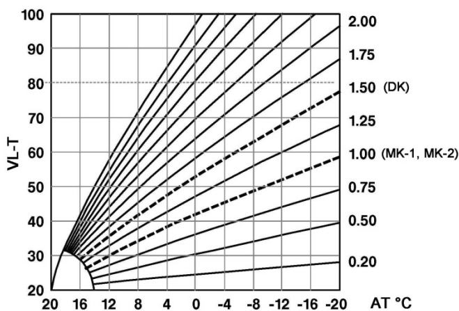
Abb. 57: Heizkennlinie (Steilheit)
