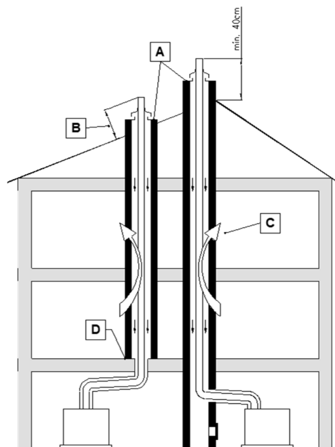
Abb. 27: Schachtqualität für Abgasleitungen
