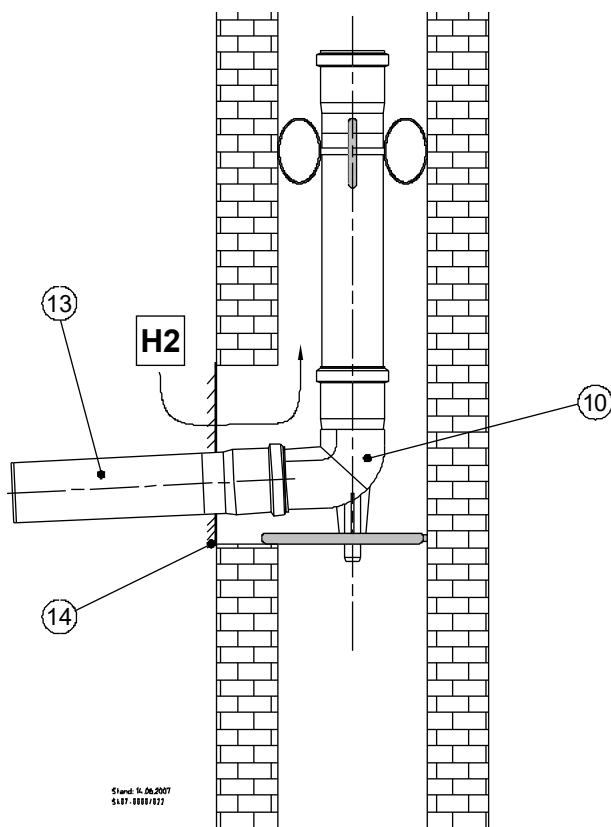
Abb. 44: Schachteinführung
