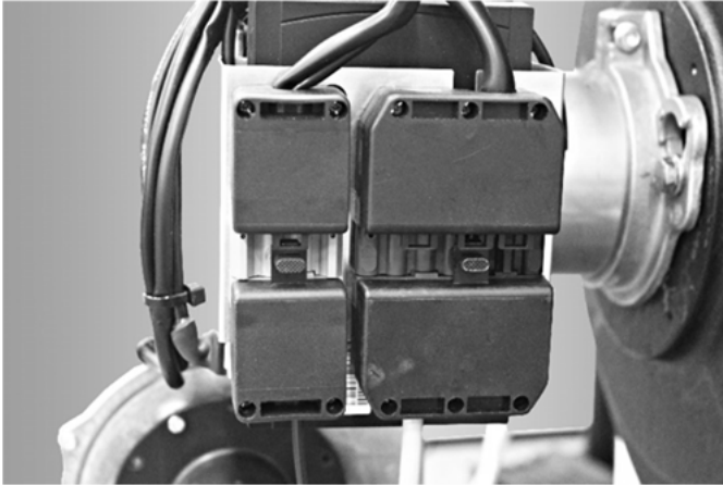
Abb. 62: Euro-Anschluss-Stecker beim RM 1 EUG (Beim RE HUG sowie beim GE HUG ist der 4-polige Euro-Anschluss-Stecker nicht enthalten.)
