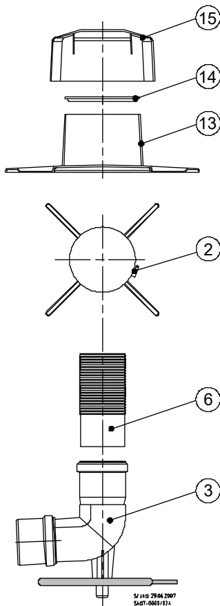
Abb. 47: Detail-Zeichnung Befestigung Schachtabdeckung
