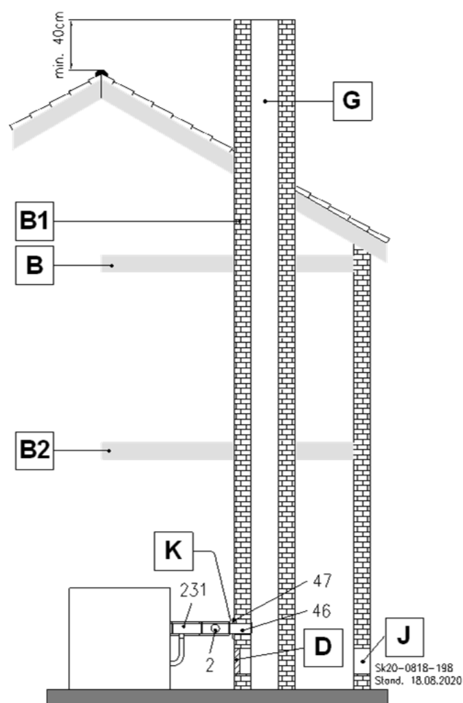
Abb. 30: B 33 Abgasrohr endet im feuchteunempfindlichen Schornstein
