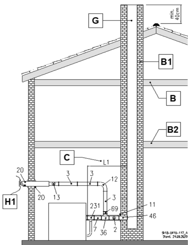
Abb. 36: C 83x Anschluss an einen feuchte-unempfindlichen Abgasschornstein und Zuluft durch die Außenwand
