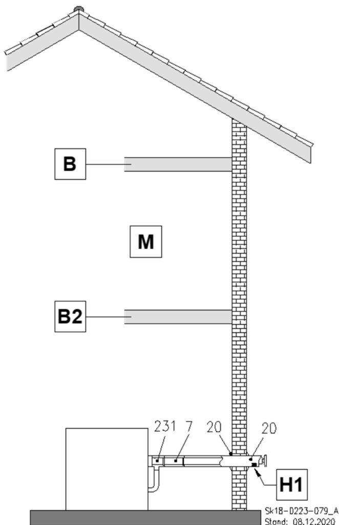
Abb. 31: C 13x Luft-Abgas-Rohrsystem horizontal durch die Außenwand
