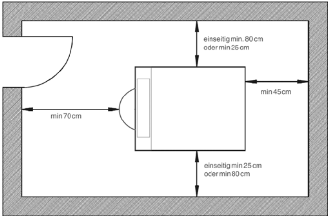
Abb. 1: Empfohlene Wandabstände
