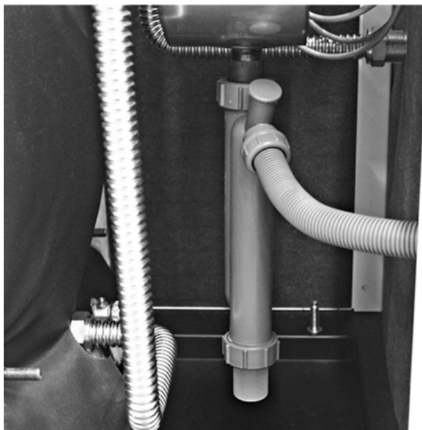
Abb. 9: Montage des Kondensatschlauchs
