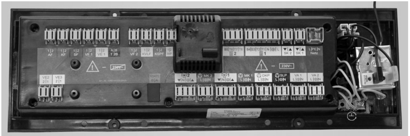
Abb. 24: Rückseite des Unit-Schaltfeldes
