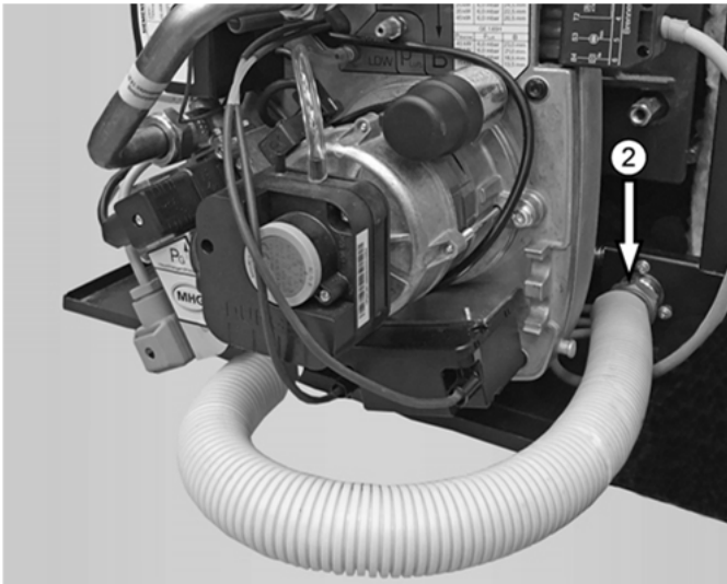
Abb. 63: Brenner-Gasanschluss ② am Kessel
