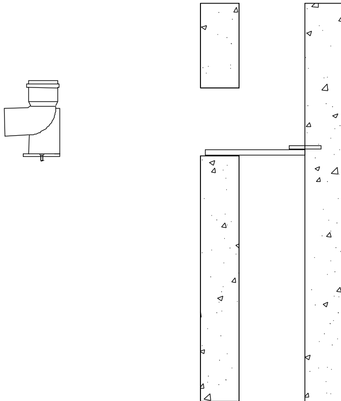
Abb. 40: 87° Stützbogen und Auflageschiene
