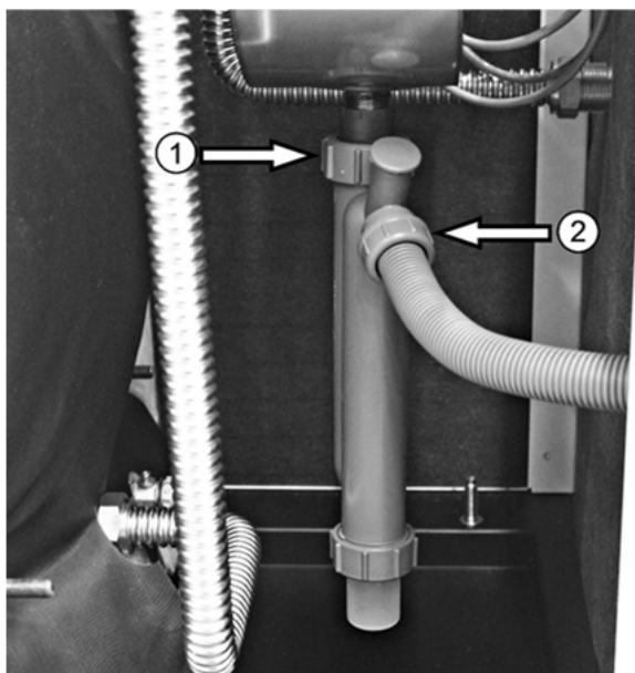
Abb. 67: Demontage des Kondensat-Siphons
