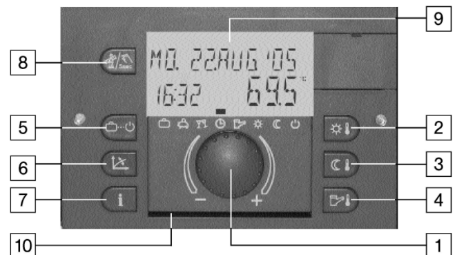
Abb. 74: Bedieneinheit
