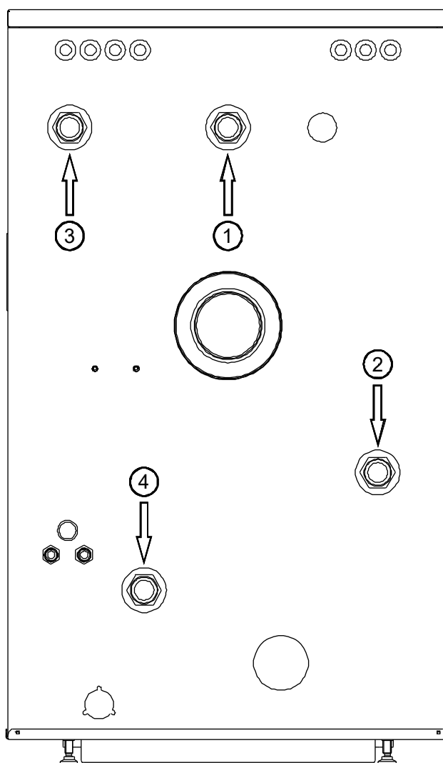
Abb. 13: Hydraulische Anschlüsse an der Kesselrückwand
