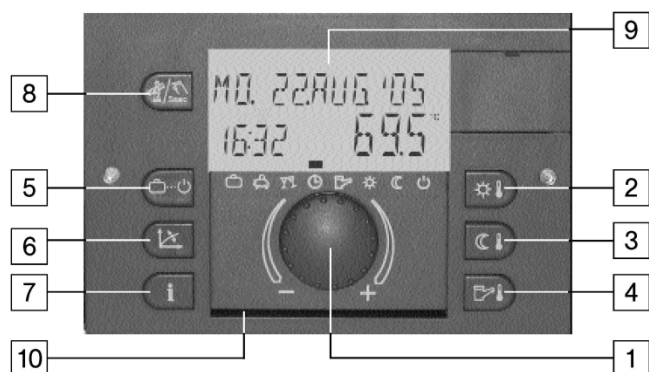
Abb. 56: Bedieneinheit
