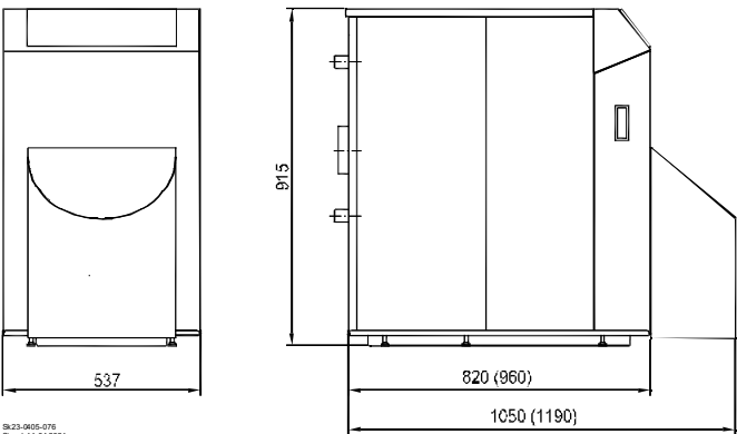
Abb. 2: Abmessungen
