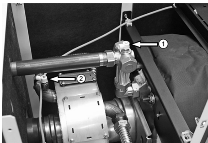
Abb. 17: Kesselkörper-Entlüfter ① sowie RWT-Entlüfter ② (bei Variante ohne interne Kreise)
