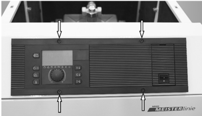
Abb. 18: Befestigungsschrauben des Unit-Schaltfeldes
