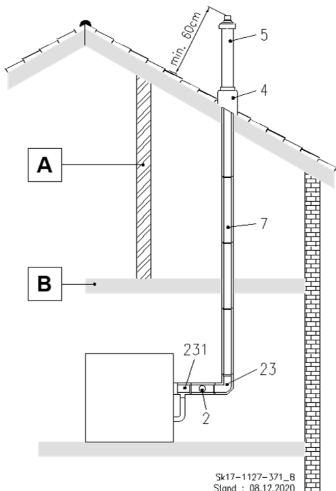
Abb. 32: C 33x Luft-Abgas-Rohrsystem senkrecht durch eine Decke und eine Dachhaut
