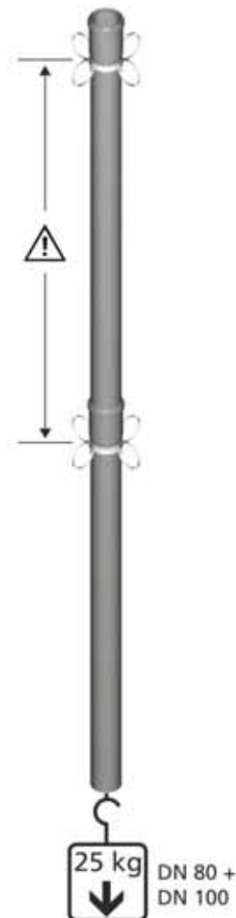
Abb. 41: Abgasrohre mit Stoppring-Technik ①
