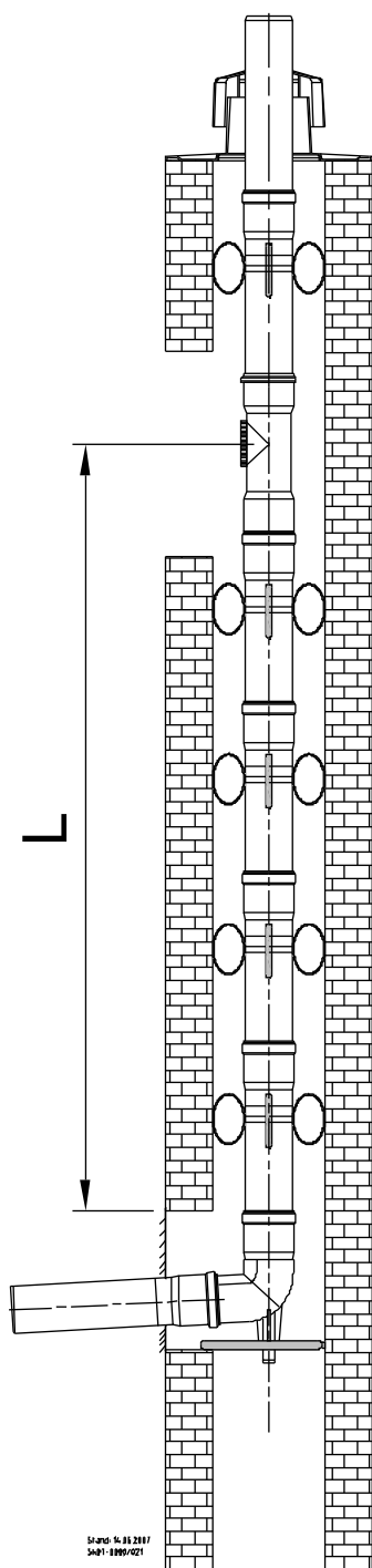
Abb. 42: Kaminsystem, starr, zur Ermittlung von Abstandsmaß L
