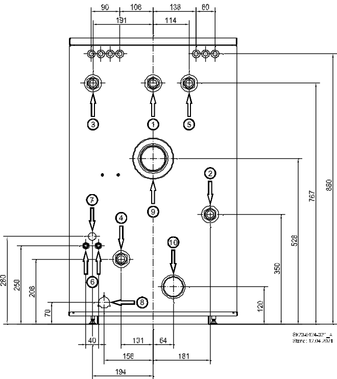
Abb. 3: Abmessungen Rückseite
