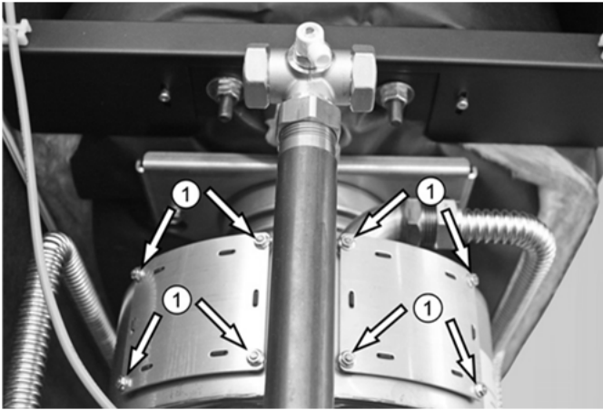
Abb. 68: Befestigungsmuttern ① der Reinigungsabdeckungen vom RWT
