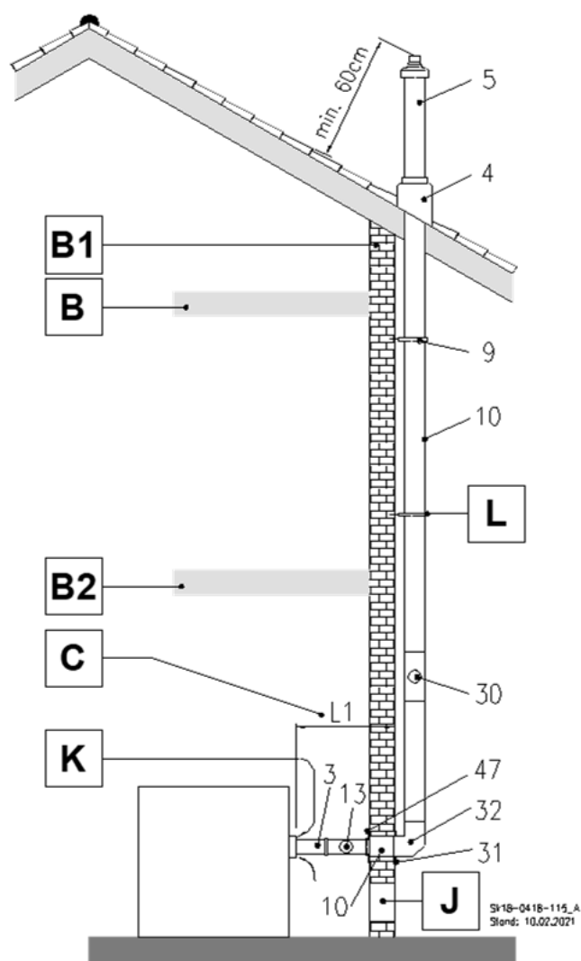
Abb. 28: B 23 Abgasrohr an der Außenwand
