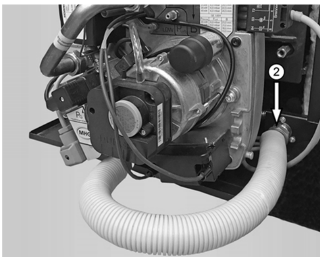
Abb. 12: Brenner-Gasanschluss ② am Kessel
