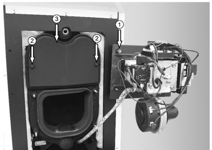
Abb. 65: Brenner-Serviceposition und Demontage der oberen Kesseltür (Der abgebildete Brenner entspricht evtl. nicht dem gelieferten.)
