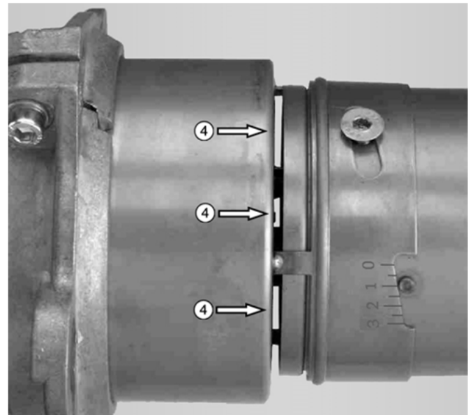
Abb. 9: Rezirkulationsschlitze ④
