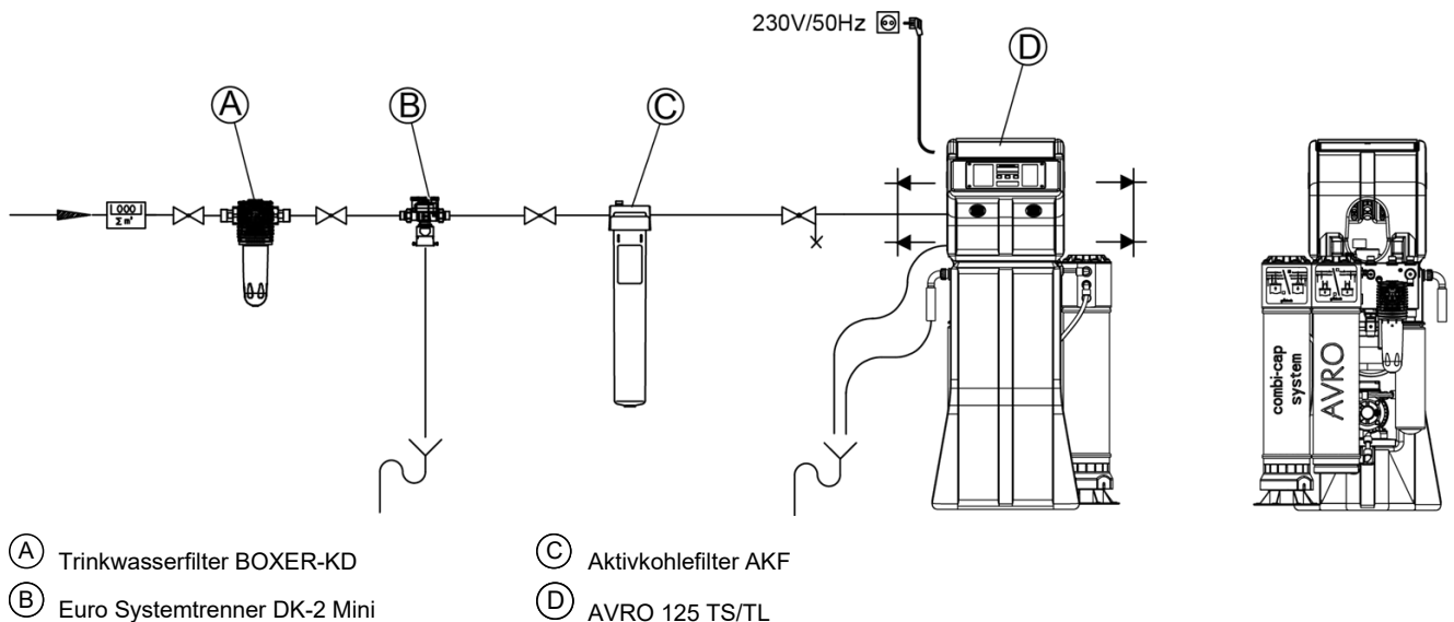
Abb. 2: Installationszeichnung
