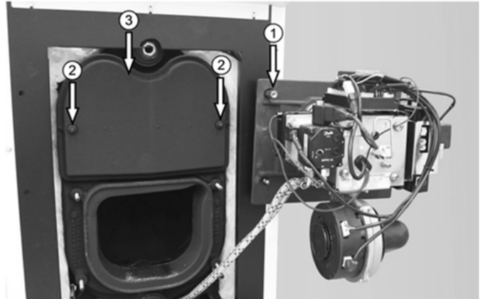
Abb. 48: Brenner-Serviceposition und Demontage der oberen Kesseltür (Der abgebildete Brenner entspricht evtl. nicht dem gelieferten.)
