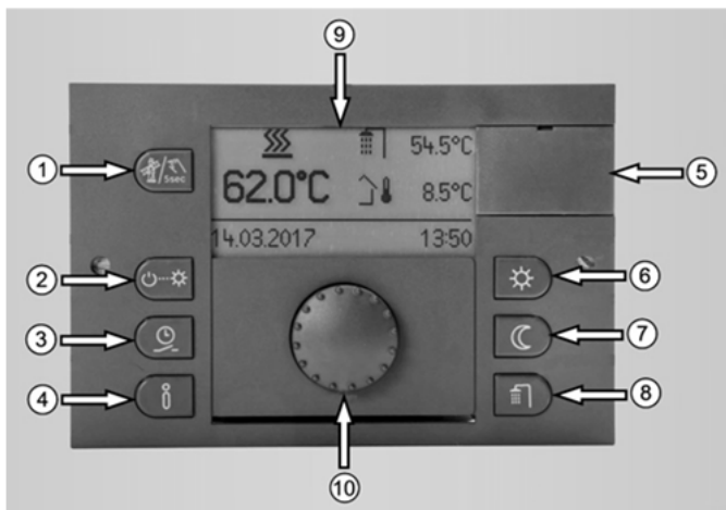
Abb. 55: Bedieneinheit
