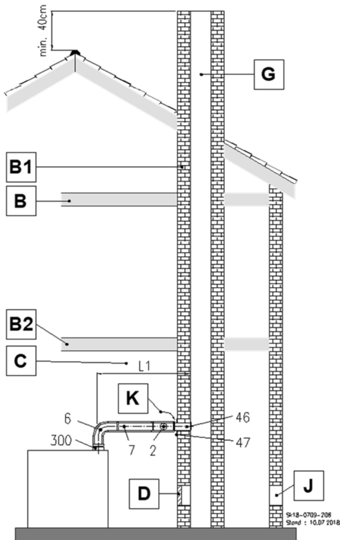
Abb. 24: B 33 Abgasrohr endet im feuchteunempfindlichen Schornstein
