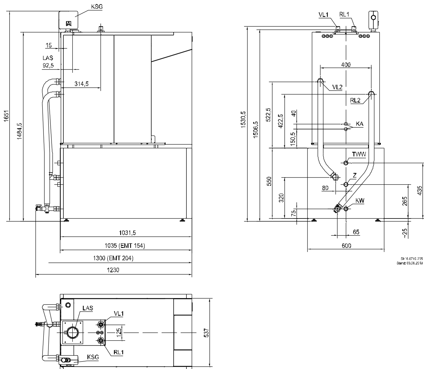
Abb. 3: Abmessungen EcoStar plus mit Trinkwarmwasserspeicher (untenliegend) THERMAT EMT-154
