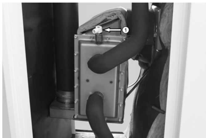
Abb. 21: Entlüfter ① des Abgaswärmetauschers
