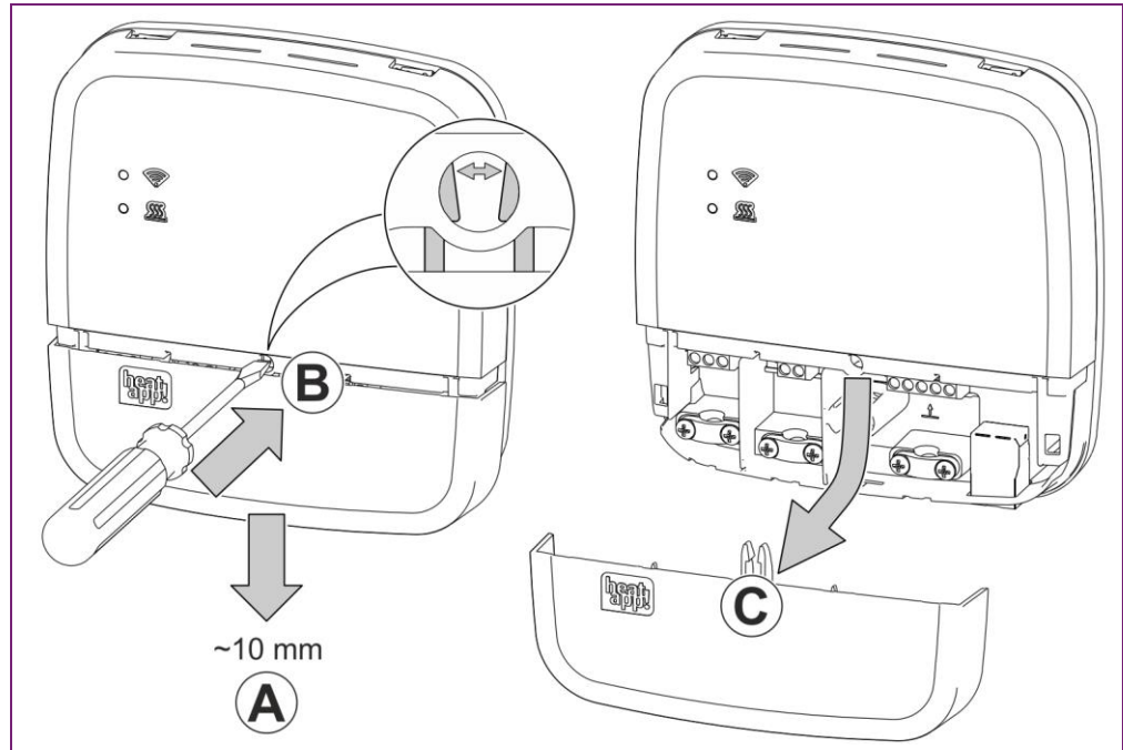
Abb. 2: Gehäuse öffnen heatapp! base
