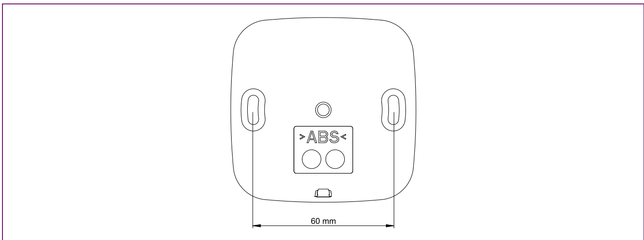
Abb. 42: Bohrbild
