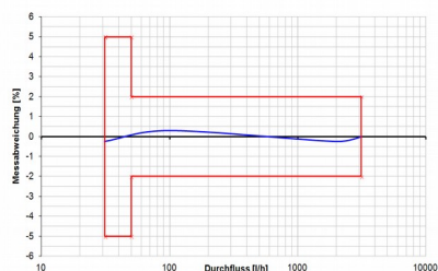
Typische Fehlerkurve für Q 3 =2,5 R80H
