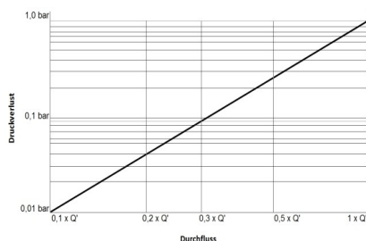
Typische Druckverlustkurve
