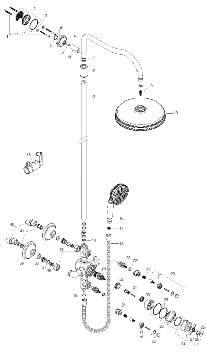
製品分解図
