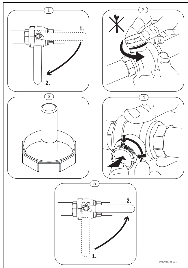
Bild 14 Siebreinigung
