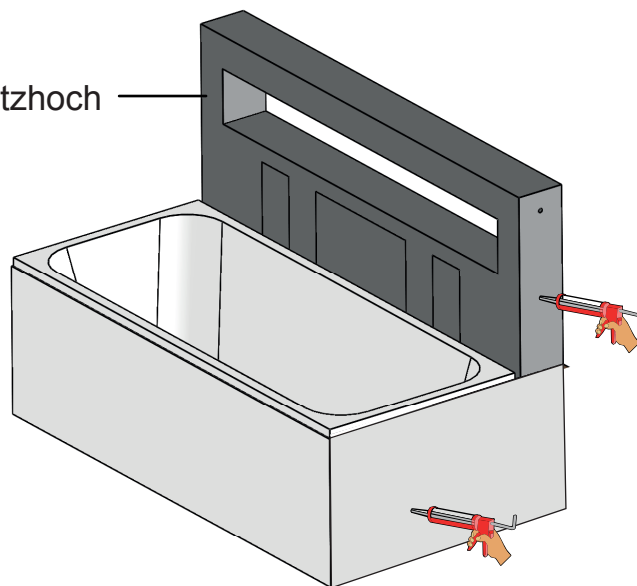
Anbaumodul Wanne sitzhoch
