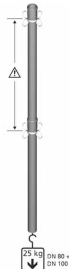
Abb. 47: Abgasrohre mit Stopping-Technik ①
