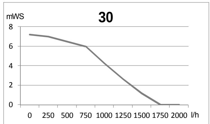
Abb. 104: Restförderhöhe ecoGAS 30, 30/36
