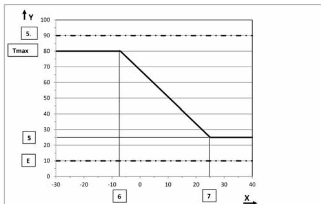
Abb. 70: Heizkennlinie gemäß Werkseinstellungen
