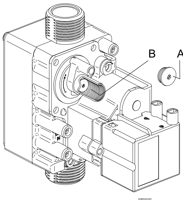
Abb. 77: Gasarmatur
