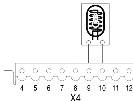
Abb. 24: Anschluss Trinkwarmwasserspeicher-Temperaturfühler
