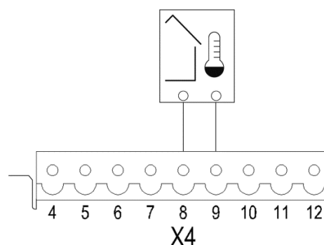
Abb. 23: Anschluss Außentemperaturfühler
