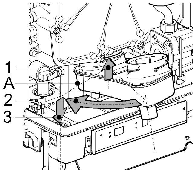
Abb. 86: Montage der Kondensatschale
