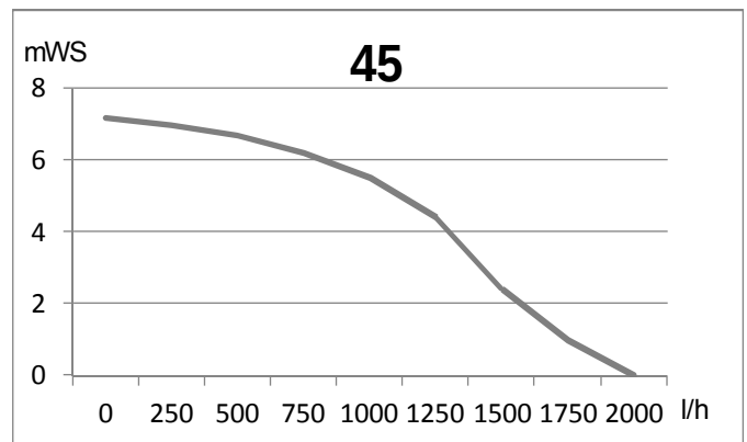
Abb. 105: Restförderhöhe ecoGAS 45, 45/36
