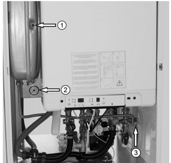
Abb. 61: Drei wichtige Stellen bei der Befüllung der Anlage (Kompakt)
