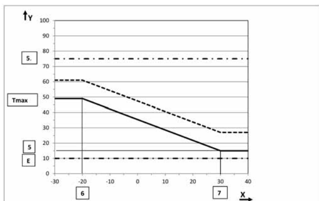
Abb. 72: Heizkennlinie mit Parallelverschiebung ( T_{\text{RaumSoll}} = 24^\circ C , r = 3 )
