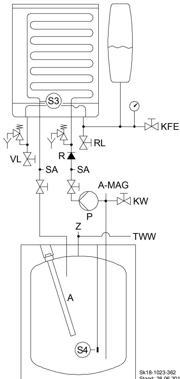
Abb. 19: Fließschema
