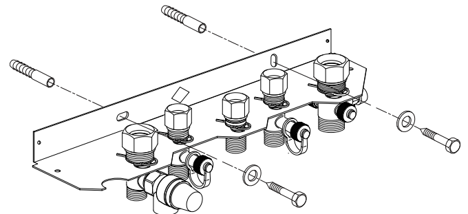
Abb. 9: Anschluss-Schiene ecoGAS Kombi
