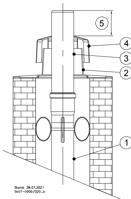
Abb. 49: Schachtabdeckung
