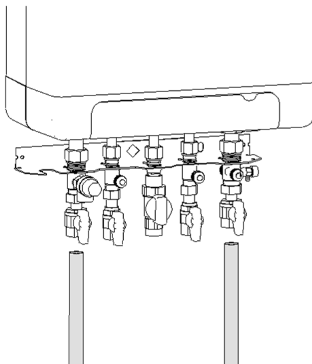
Abb. 14: Montage Vorlauf- und Rücklaufrohr
