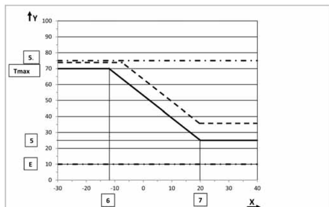
Abb. 73: Heizkennlinie mit Parallelverschiebung ( T_{\text{RaumSoll}} = 24^\circ C , r = 3 ) und Begrenzung durch Parameter „5.“
