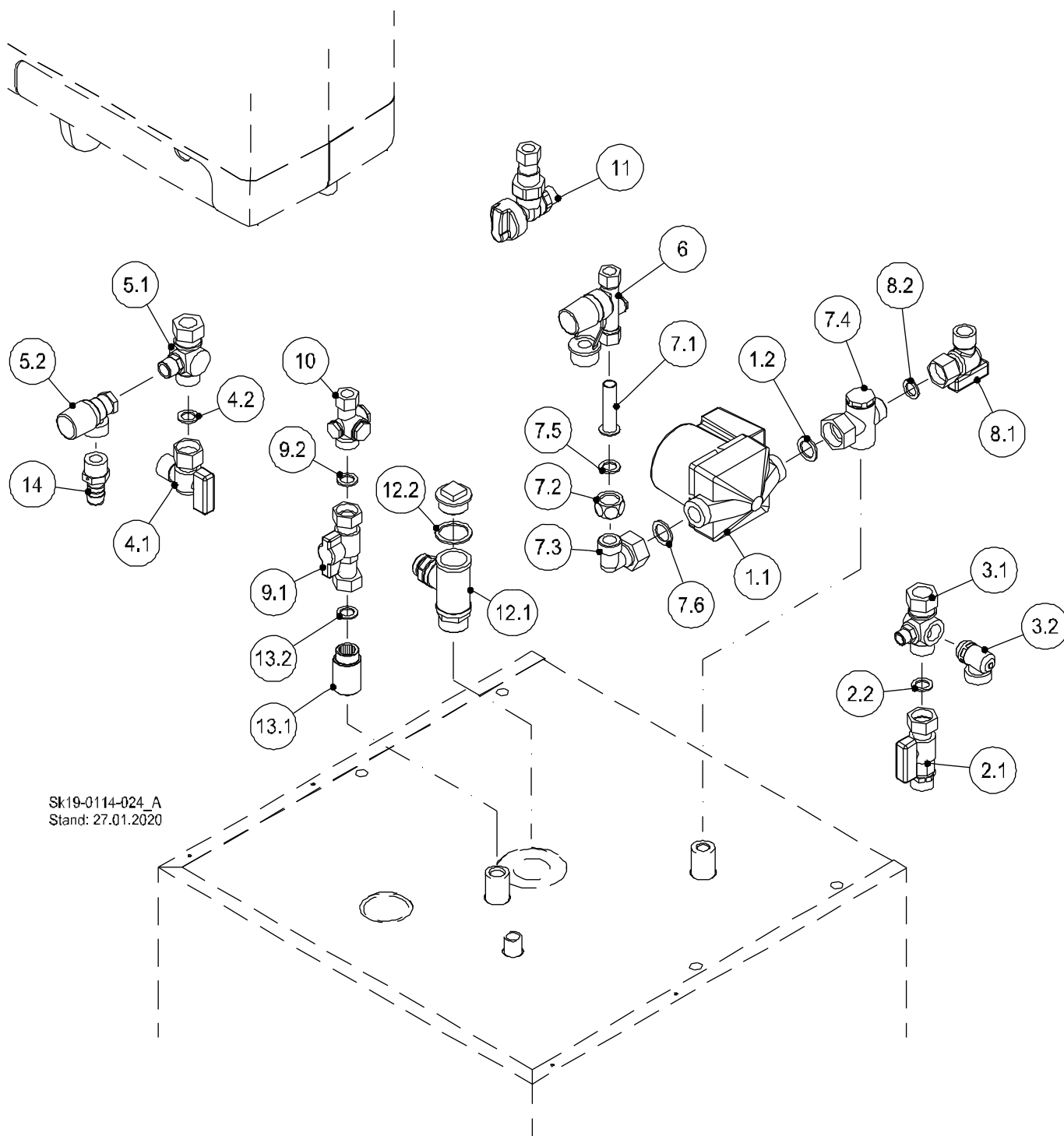
Abb. 98: Hydraulik ecoGAS Kompakt
