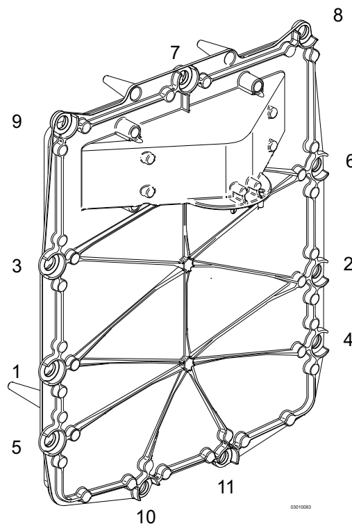
Abb. 85: Reihenfolge für das Anziehen der Pass-Schrauben
