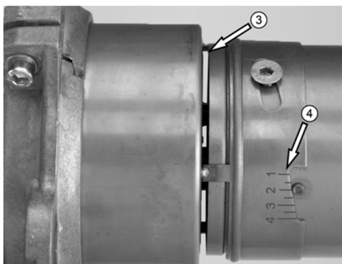
Abb. 8: Rezirkulationsschlitz (3) und Skala (4) zur Einstellung von Maß R
