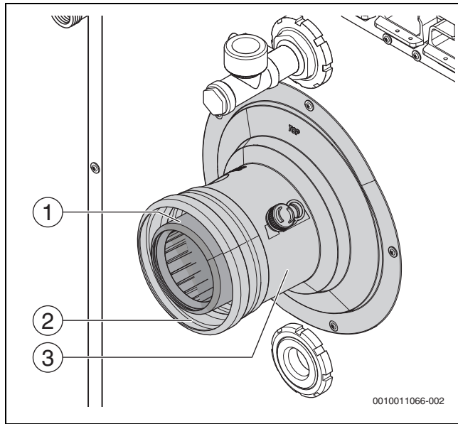
Bild 18 Abgasanschluss montieren
