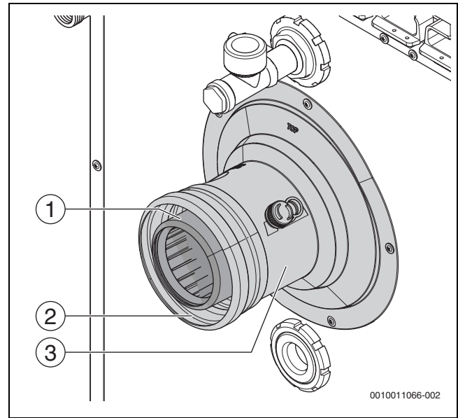
Bild 19 Abgasanschluss montieren
