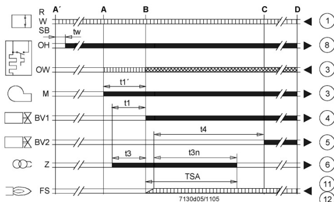
Abb. 14: Programmablauf LMO 44
