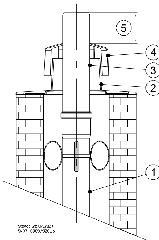
Abb. 49: Schachtabdeckung
