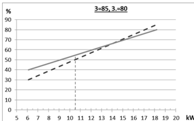
Abb. 65: Heizleistung und Pumpendrehzahl am Beispiel ecoGAS 18 mit Werkseinstellung für Parameter 3 (= 85) und Parameter 3. (= 80)
