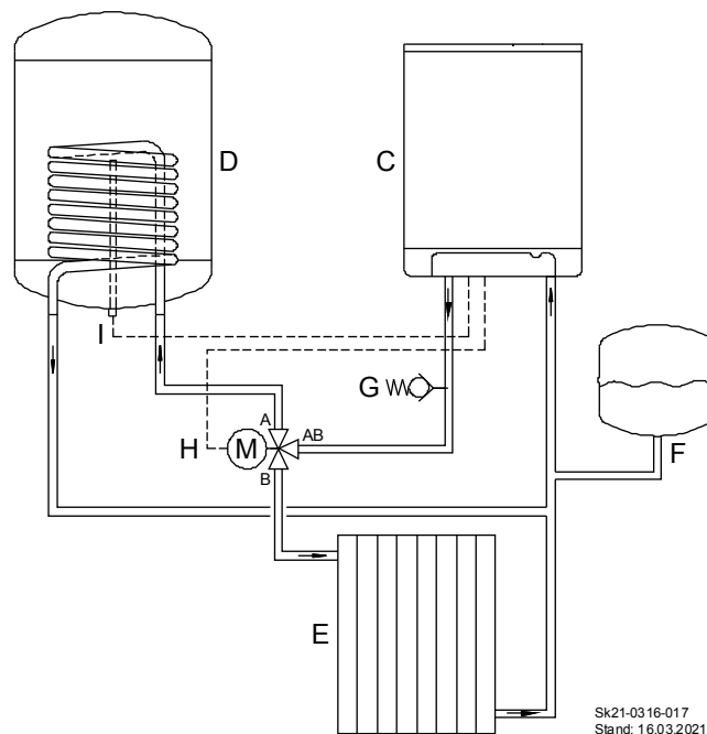
Abb. 27: Trinkwarmwasserbereitung mit externem Speicher über 3-Wege-Umschaltventil
