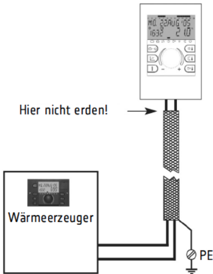
Bild 4: Einseitige Erdung der Abschirmung
