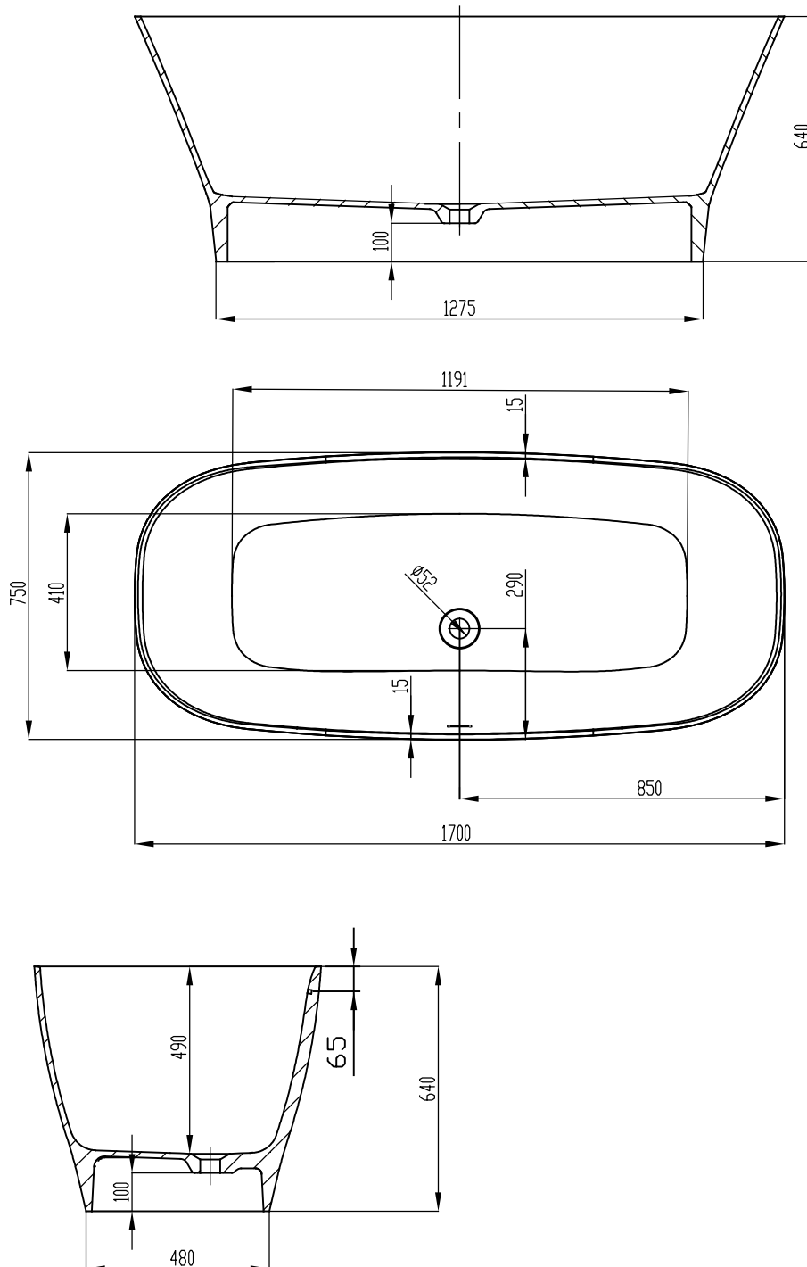
FORMAT Design Mineralgusswanne freistehend, 1700x750 Art.-Nr.1373
