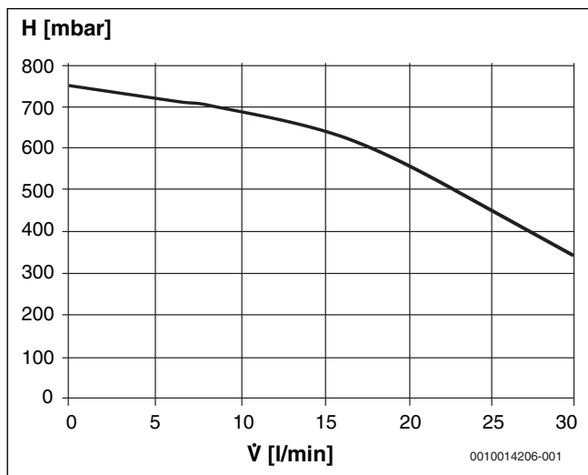
Bild 6 Restförderhöhe Primärkreispumpe
