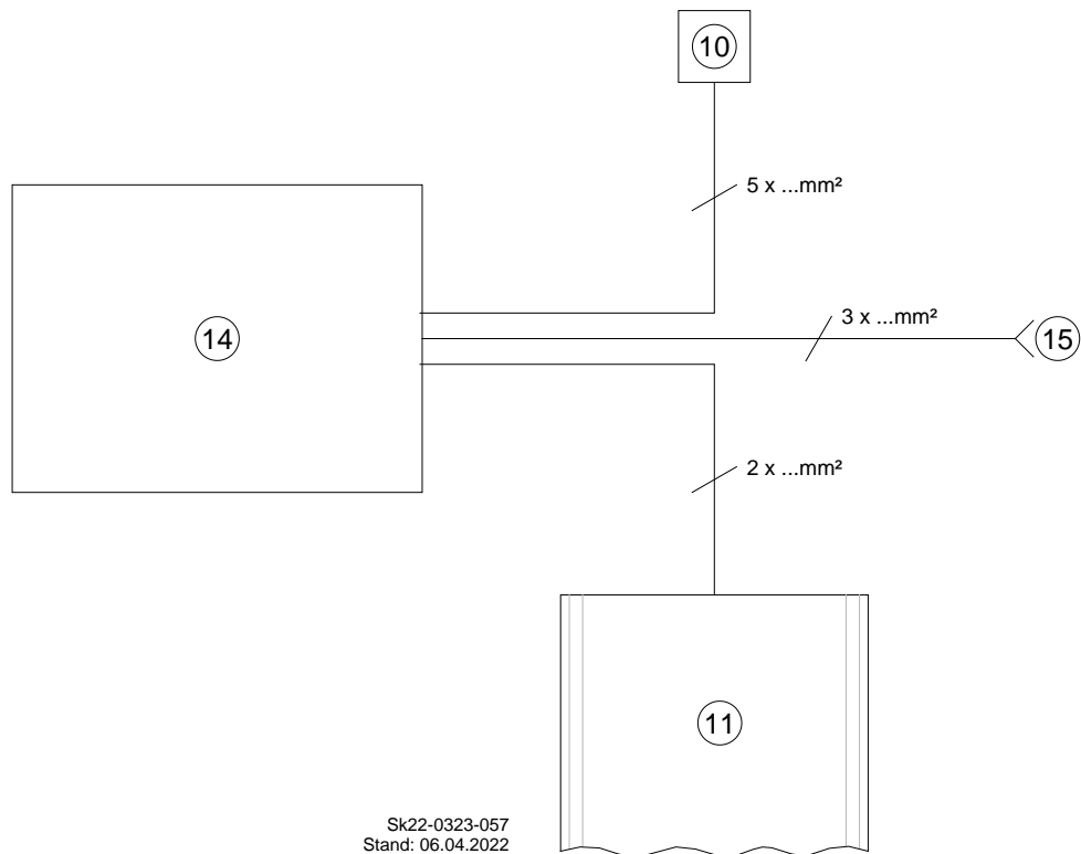
Abb. 16: Anschlussplan für Ausführung 400-1200 VA
