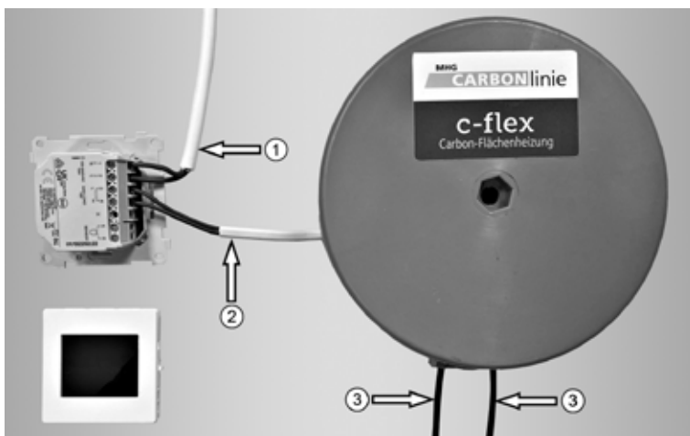
Abb. 12: Anschluss Transformator c-300 an Touch-Thermostat
