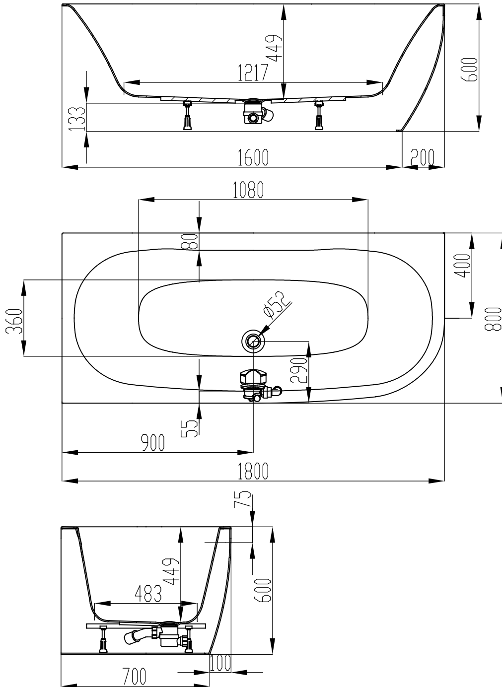
Format Design Monoblock Oval-Badewanne, 1800x800 Ecke links mit Überlaufbefüllung Art.-Nr.1385
