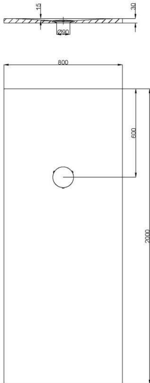
Duschwannen Nias 2000x800 Rechteck 4560xA ungeschnitten
