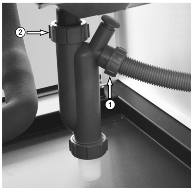
Abb. 50: Demontage des Kondensat-Siphons
