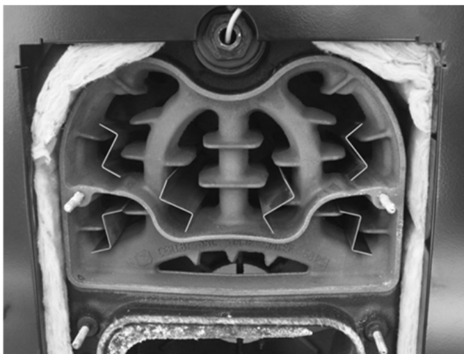
Abb. 49: Geöffneter Kessel
