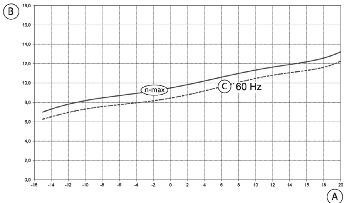
Abb. 59: Heizleistung ecoWP 15Xe bei Vorlauftemperatur 45°C
