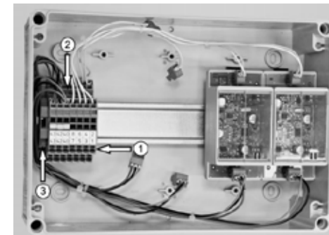
Abb. 2 Wandgehäuse mit Kabelbaum und Kaskadenmodulen
