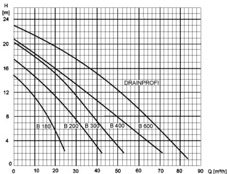
Kennlinien (bei 2850 min -1 )
