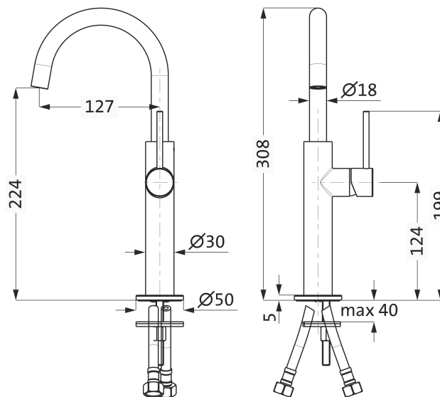
Lochbohrung 35mm
