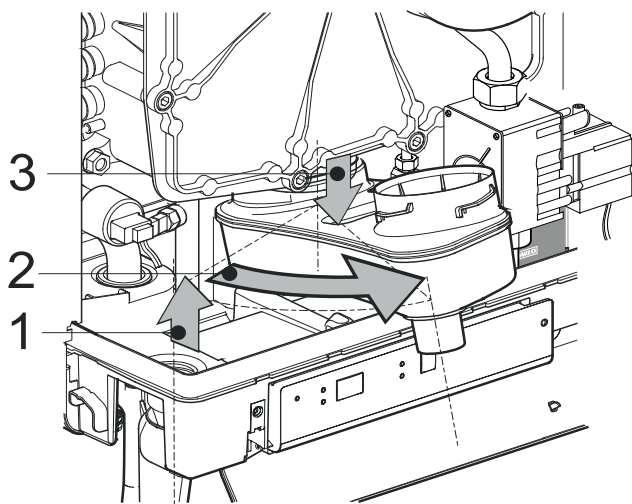
Abb. 80: Demontage Kondensatschale
