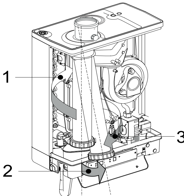
Abb. 79: Demontage Abgasrohr
