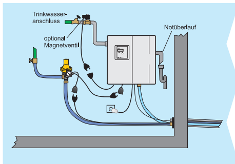
Installationsschema mit Unterwasserpumpe COMBIPRESS
