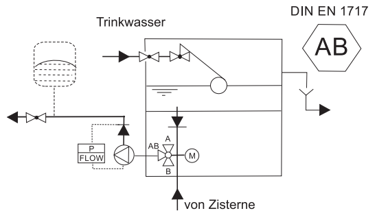
Installationsschema mit CPS Hauswasserwerk
