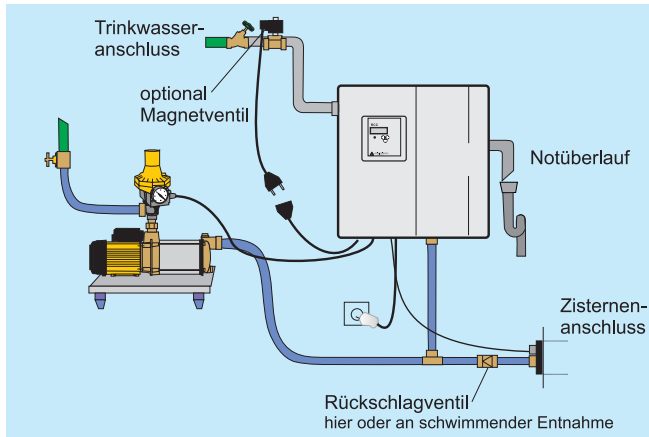
Installationschema mit CPS Hauswasserwerk
