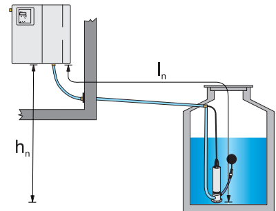
vereinfachtes Bild: ausführliches Installationsschema ↪ Kap. 5.4 „Anschluss einer Unterwasserpumpe COMBIPRESS“
