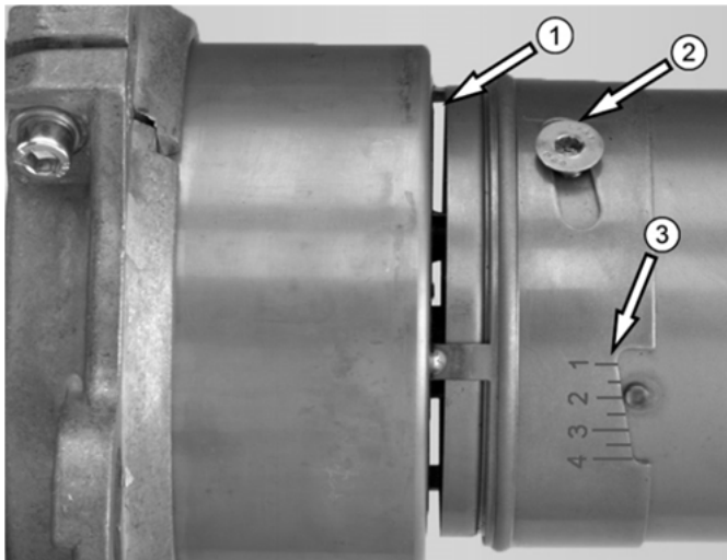
Abb. 32: Rezirkulationsschlitze ①, Befestigungsschraube ② und Skala ③
