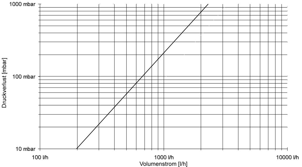
Bild 2: Widerstandsdiagramm
