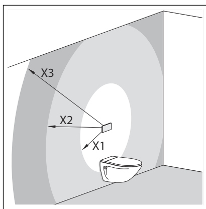
Abb. 9: Einbauort des Netzteils
