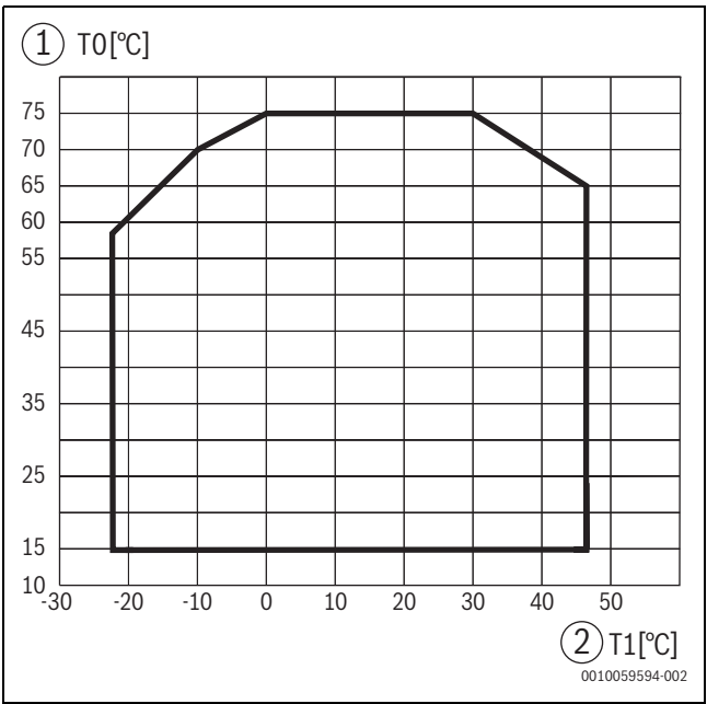
Bild 4 Wärmepumpe im Heizbetrieb ohne Zuheizer
