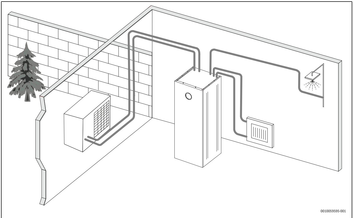
Bild 7 Außeneinheit, Inneneinheit mit Zuheizer und Warmwasserspeicher CS3800iAW O-S / CS3800iAW O-T
