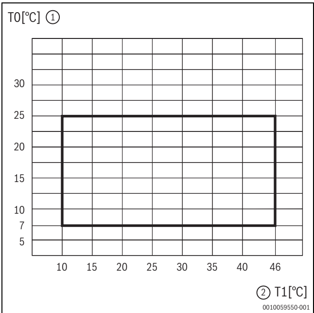
Bild 5 Wärmepumpe im Kühlbetrieb
