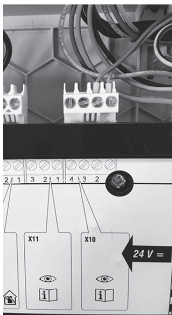
Abb. 5: Anschlussklemme X10
