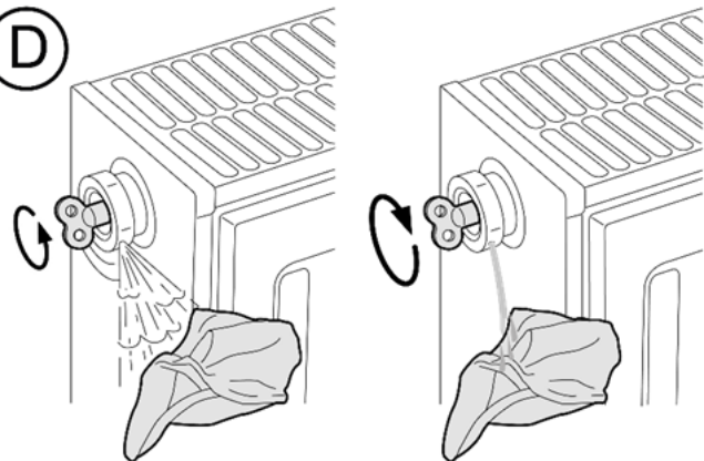
Abb. 10: Entlüftung der Heizkörper
