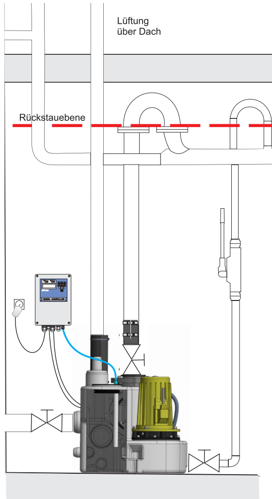
Anwendung mit einer Hebeanlage
