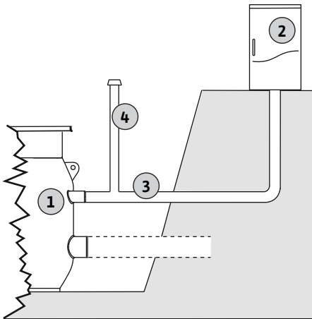
Fig. 5: Installationsbeispiel für Pumpenschacht und Schaltschrank
