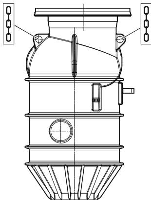
Fig. 4: Anschlagpunkte
