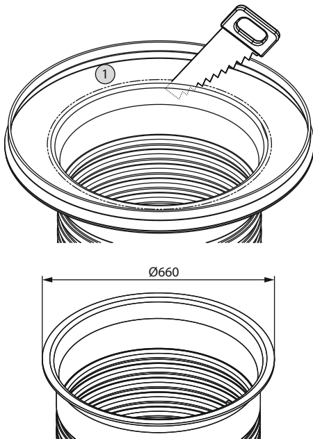
Fig. 10: Deckelflansch ausbauen
