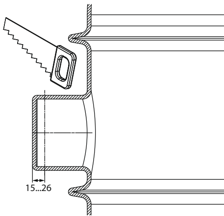
Fig. 7: Vorbereitung der Rohranschlüsse
