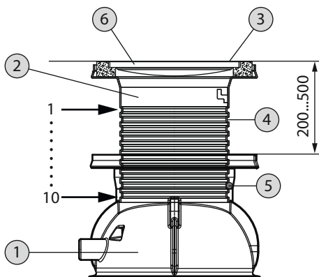
Fig. 8: Installation Schachtverlängerung
