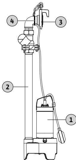
Fig. 14: Pumpe montieren
