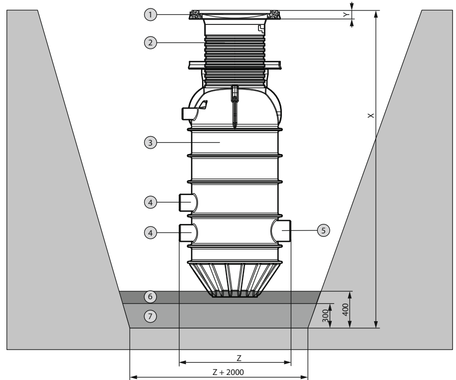
Fig. 6: Installation des Pumpenschachts
