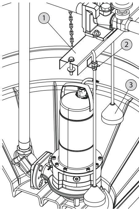
Fig. 15: Anbringen der Signalgeber
