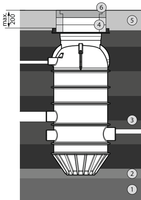
Fig. 11: Grubenbefüllung (mit installierten Schachtabdeckungen vom Typ A15 und B125)
