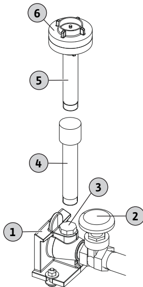
Fig. 17: Spülanschluss montieren
