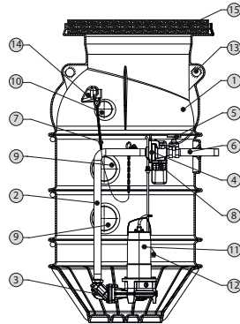
Fig. 1: Übersicht
