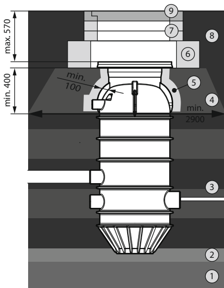
Fig. 12: Grubenbefüllung (mit installierter Schachtabdeckung vom Typ D400)
