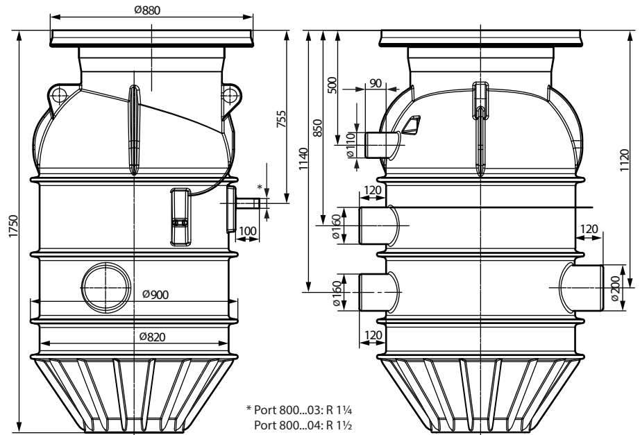
Fig. 2: Maßzeichnungen 1750 mm
