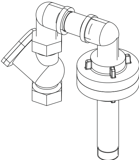
Fig. 18: Vakuumbrecher montieren
