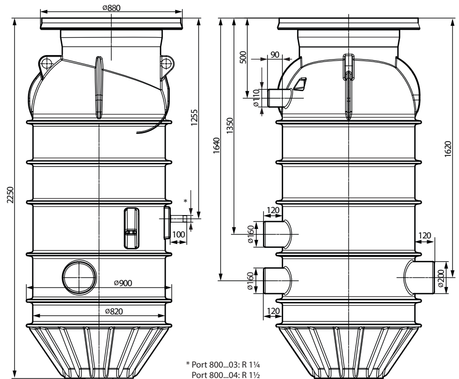
Fig. 3: Maßzeichnungen 2250 mm
