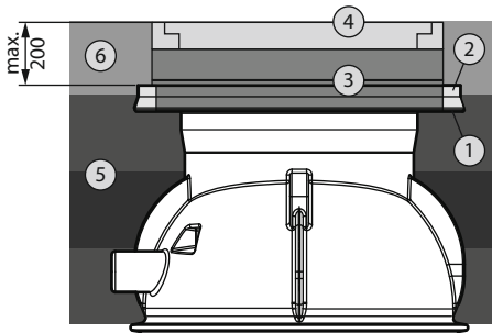
Fig. 9: Anbringen der Betonringe zum Höhenausgleich
