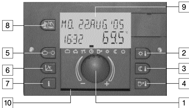
Zentralgerät
