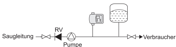
Trockenaufgestellte Pumpe
