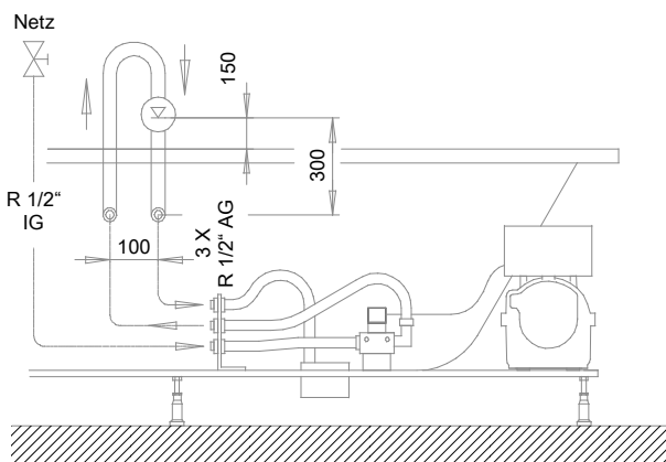
Einheit für Nach-/Zwischenspülung Wannenseitig vorinstalliert
