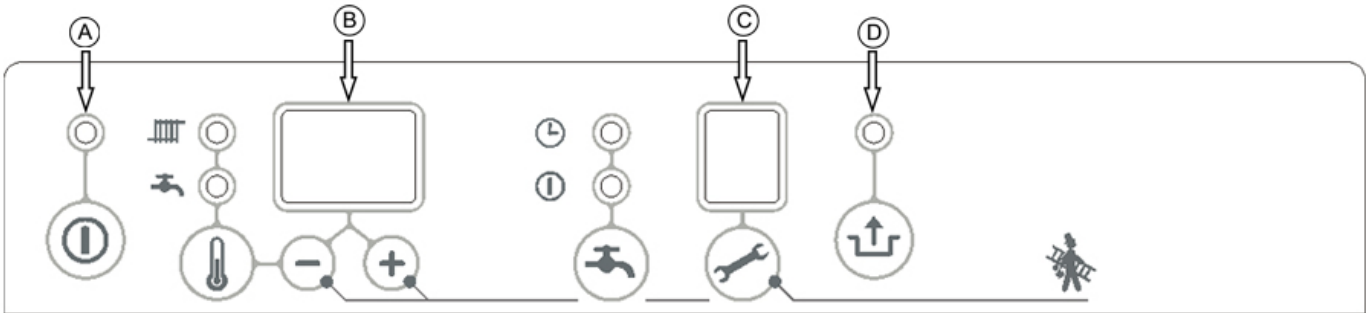
Abb. 2: Bedienfeld
