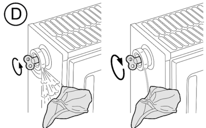
Abb. 55: Entlüftung der Heizkörper
