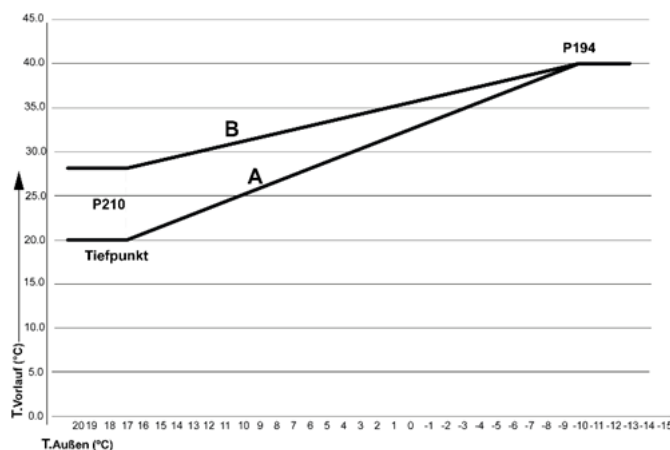
Abb. 50: Heizkennlinie (T.Vorlauf gegen T.Außen)
