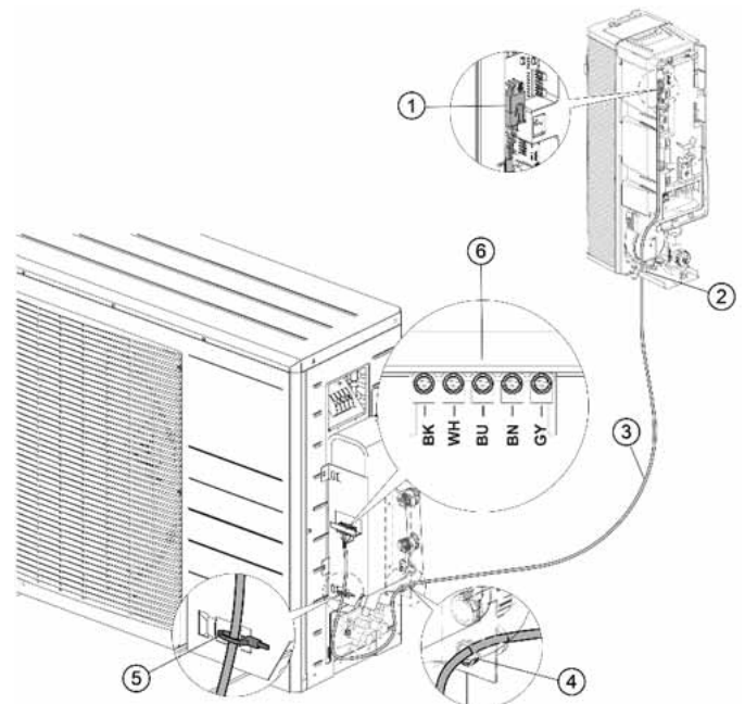
Abb. 25: Befestigung der Drähte an der Fühlerklemmleiste ⑥
