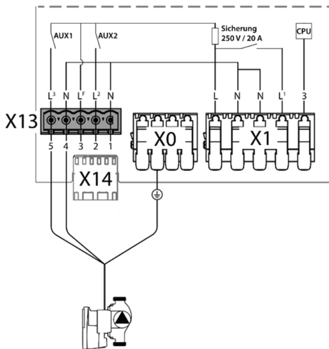
Abb. 32: Anschluss einer externen Heizkreispumpe
