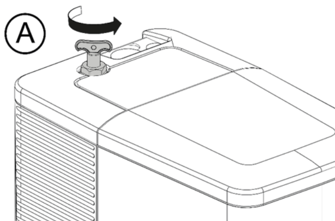
Abb. 17: Manueller Entlüfter A der Inneneinheit
