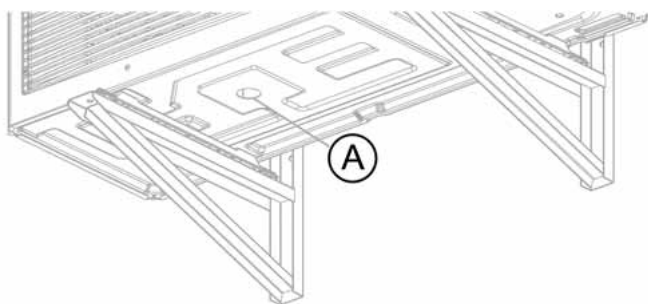
Abb. 9: Kondensatablauf (A) der Außeneinheit
