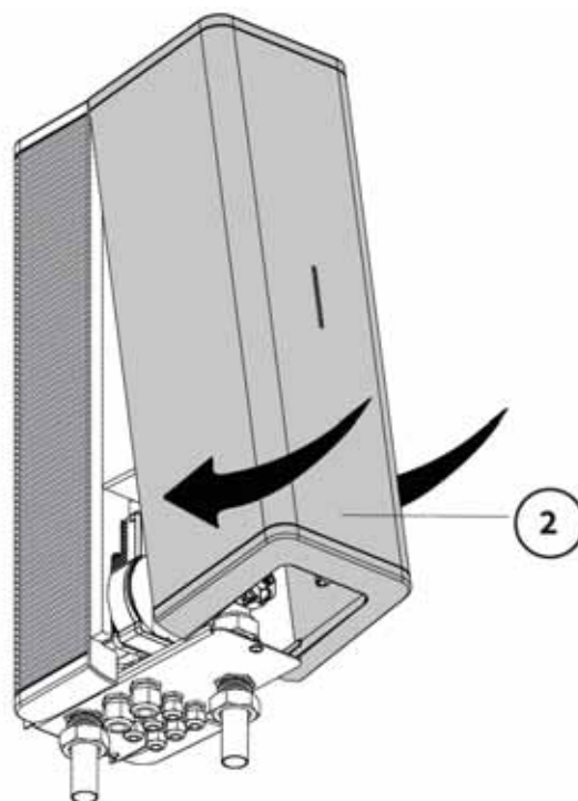
Abb. 58: Montage der Fronthaube
