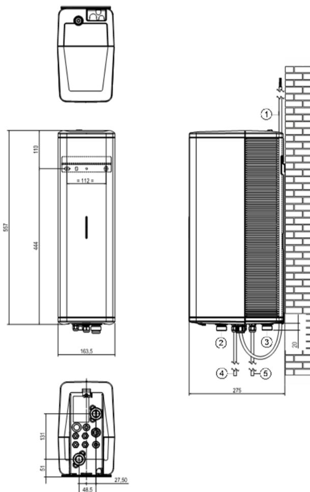
Abb. 5: Abmessungen und Anschlüsse Inneneinheit
