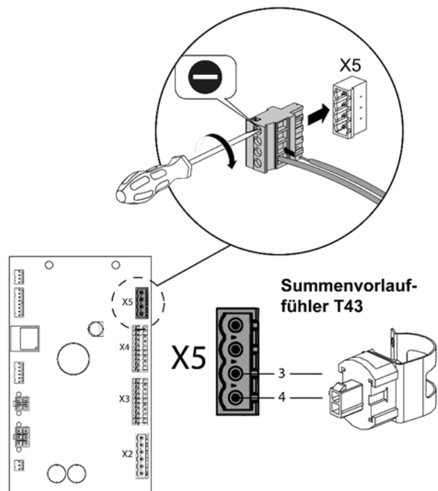
Abb. 31: Anschluss des Summenvorlauftfühlers T43
