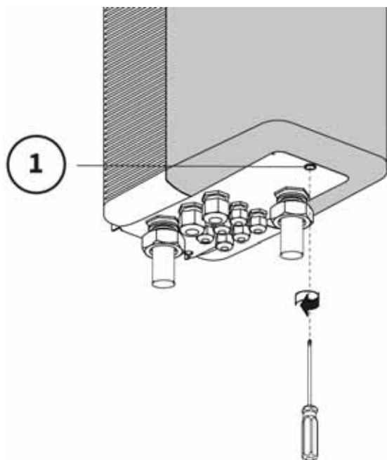
Abb. 56: Lösen der Schraube
