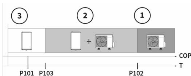
Abb. 48: Mögliche Hybridbetriebe
