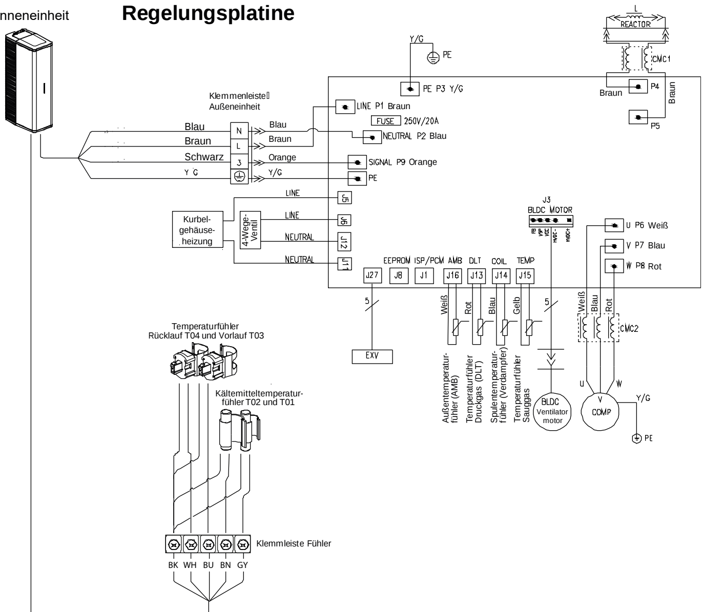
Abb. 34: Schaltplan Außeneinheit
