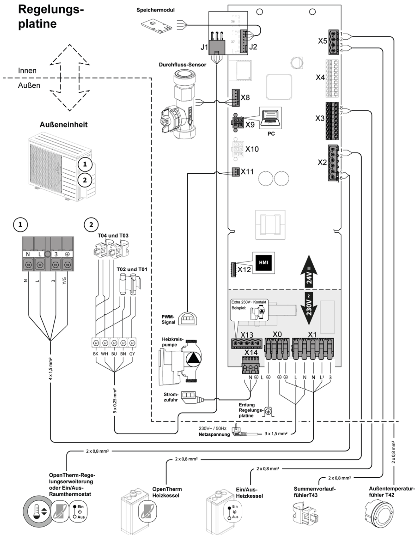
Abb. 35: Elektrischer Schaltplan Inneneinheit 30/80
