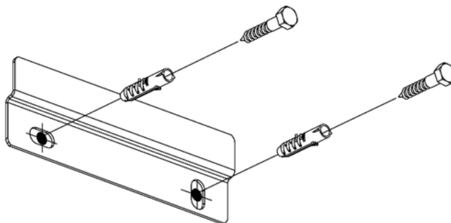
Abb. 10: Montage der Wandschiene
