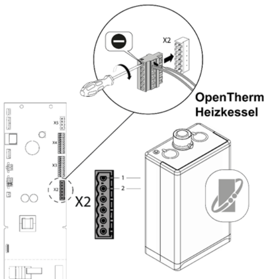
Abb. 27: Anschluss eines OpenTherm-Heizkessels
