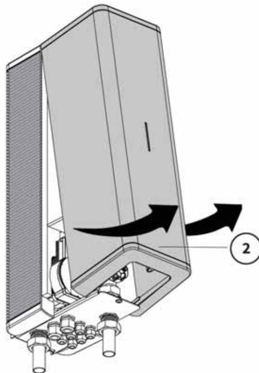
Abb. 22: Demontage der Fronthaube
