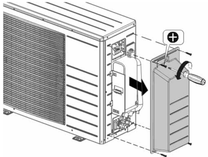
Abb. 15: Demontage Seitenverkleidung
