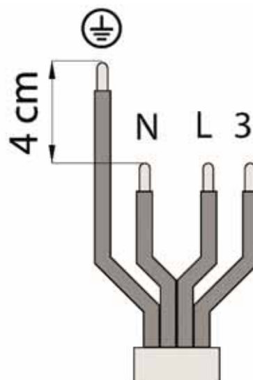
Abb. 23: Kürzung der Drähte N, L und 3
