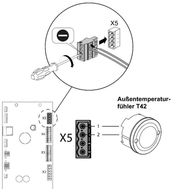
Abb. 30: Anschluss des externen Außentemperaturfühlers
