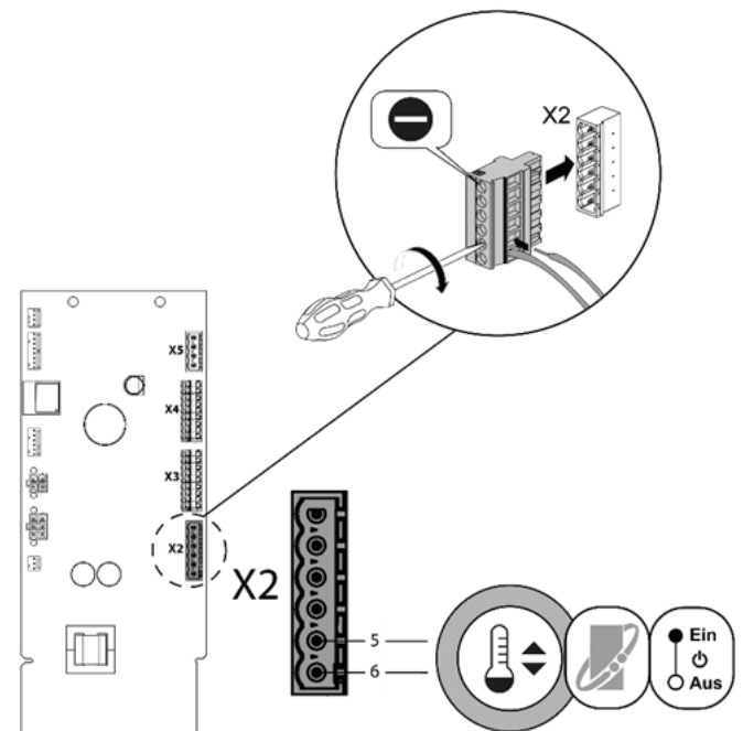
Abb. 29: Anschluss OpenTherm-Regelungserweiterung oder Ein/Aus-Raumthermostat
