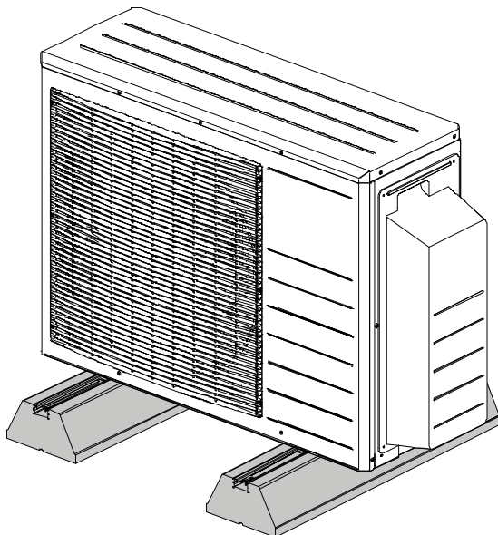
Abb. 7: Aufstellung auf Fußstützen
