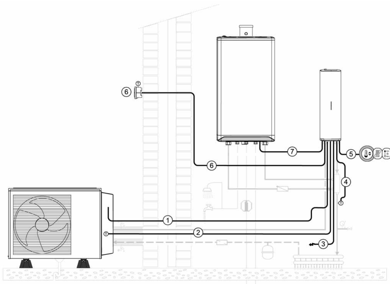
Abb. 33: Elektrische Installationsübersicht
