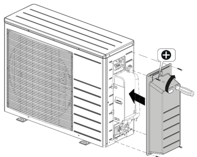
Abb. 26: Montage der Seitenverkleidung
