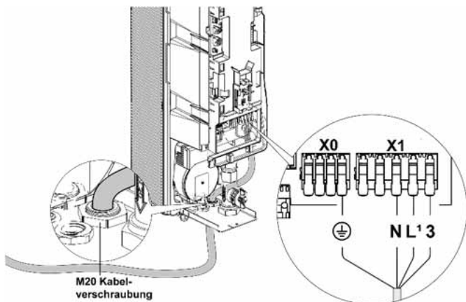
Abb. 24: Kabelführung und Kabelanschluss Inneneinheit
