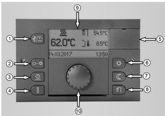
Abb. 55: Bedieneinheit
