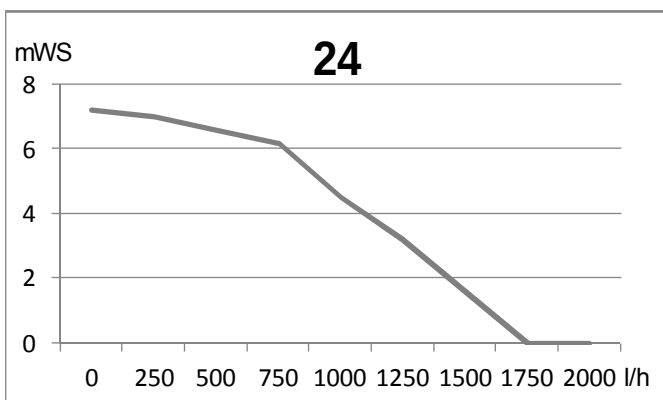
Abb. 103: Restförderhöhe ecoGAS 24, 24/28
