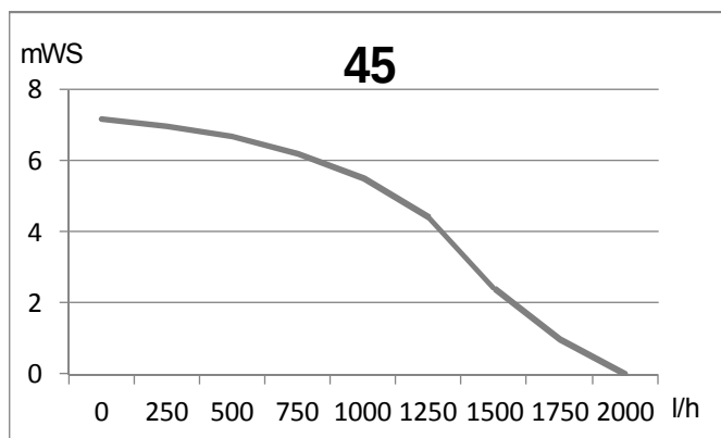
Abb. 105: Restförderhöhe ecoGAS 45, 45/36
