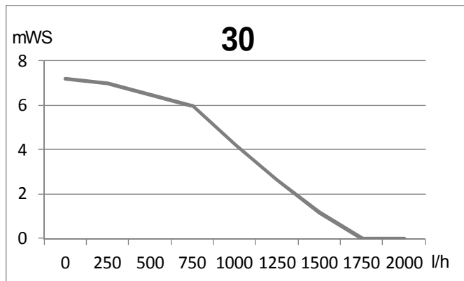
Abb. 104: Restförderhöhe ecoGAS 30, 30/36
