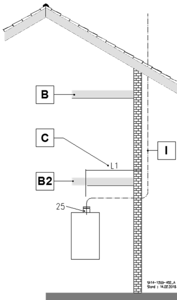
Abb. 41: C 63x Für Anschluss an eine nicht mit der Gasfeuerstätte geprüfte Verbrennungsluftzuführung und Abgasabführung
