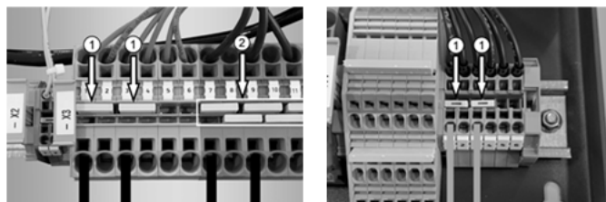
Abb. 9: Beispiel neu gesetzter Brücken
