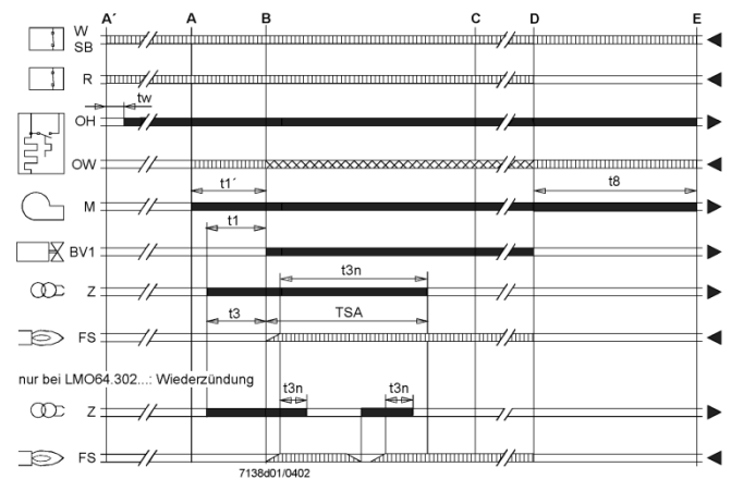
Abb. 19: Programmablauf LMO 64.301
