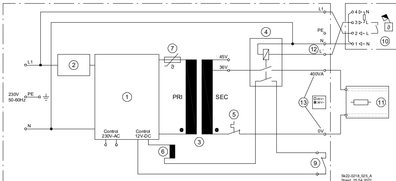
Abb. 16: Stromlaufplan – Ausführung für 2400-3200 VA
